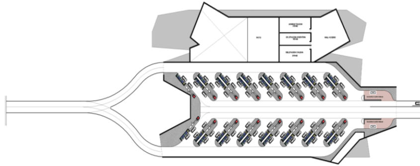
PLANTA NIVEL +8.00 CONTROL VEHICULO LIVIANO ESC 1/750
