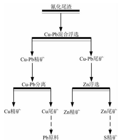
图 5 氰化尾渣中有价元素回收原则流程 [48]
