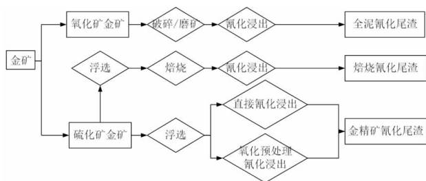
图 1 氰化尾渣的来源与分类
