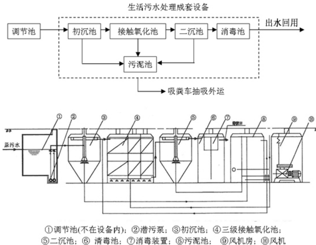
图 6.2.1-7 成套污水处理设备工艺流程图
