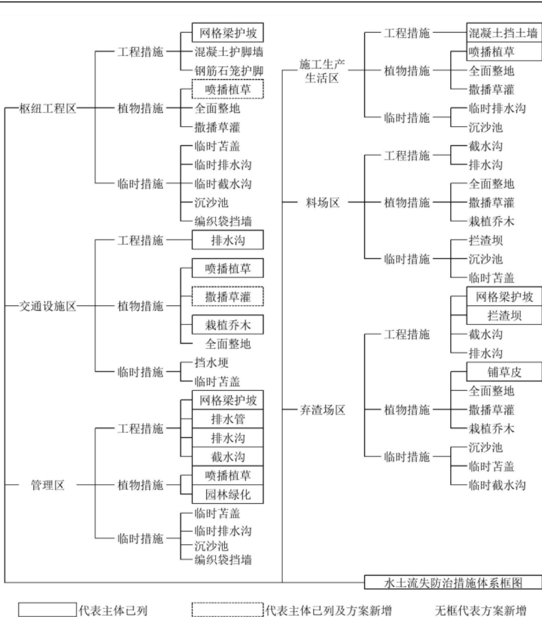
图 6.9.2.1 水土流失防治措施体系框图
