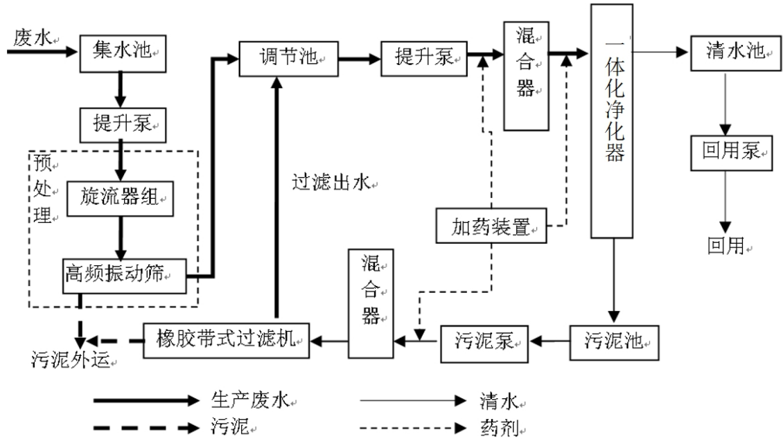
图 6.2.1-3 高效(旋流)污水净化法工艺流程图
