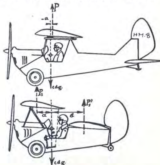
Øverst en Flyvemaskine af sædvanlig Type Nederst „Pou«en» med de to Bæreplaner, der giver større Frihed i Valget af Tyngdepunktets Bølggenhed.
