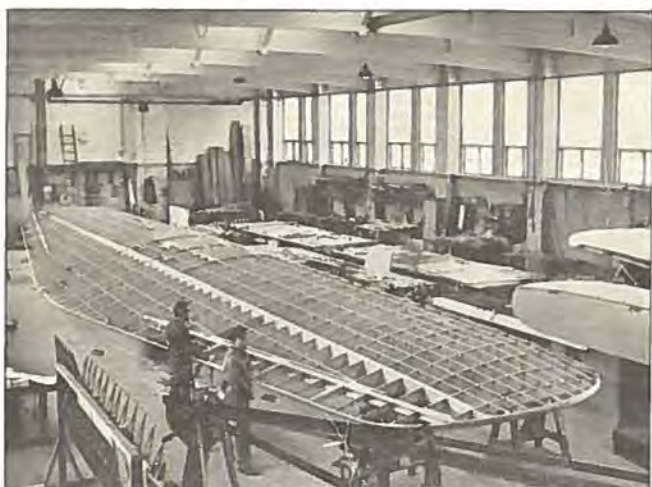
1 / 2 — Den færdige Plankonstruktion.
