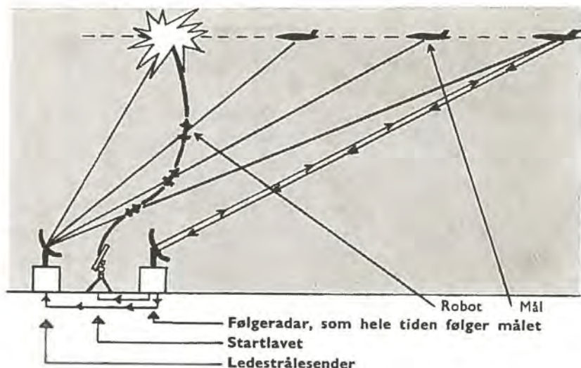
Skematisk tegning af radarfølgning og nedskydning af fly med luftværnsraketter.
