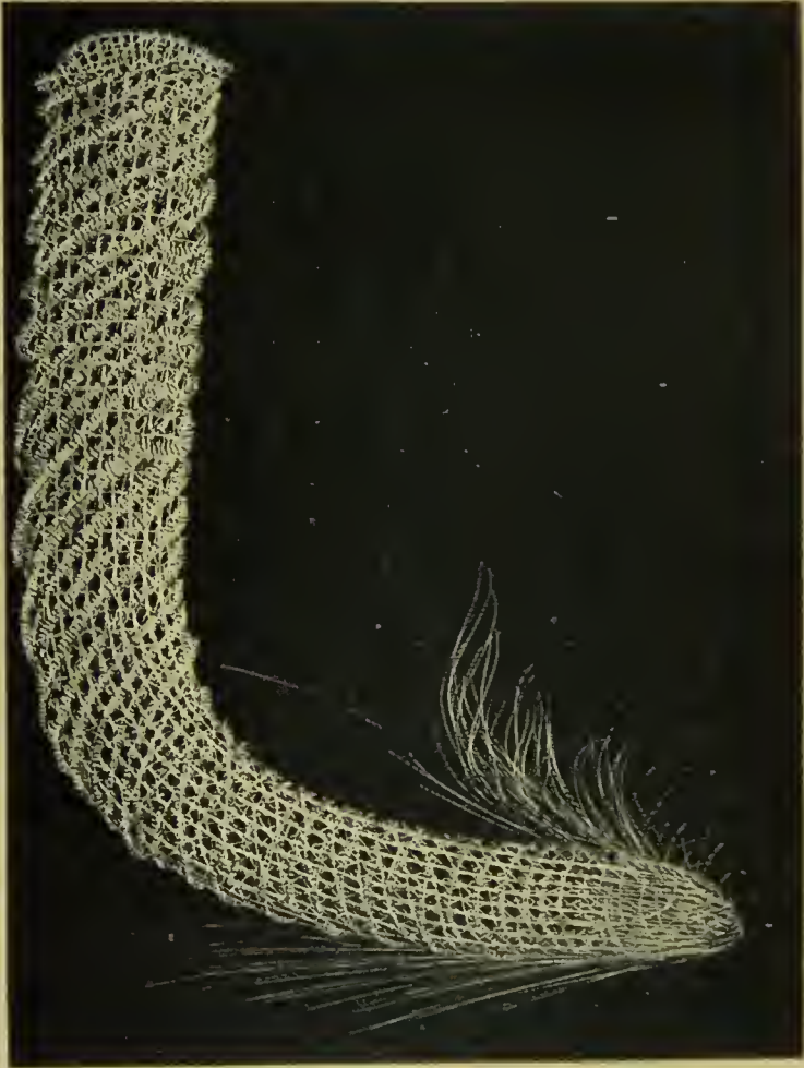
Fig. 2.— Euplectella speciosa .
