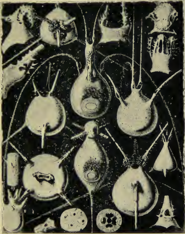
Fig. 19.—Radiolaria (Tuscarora).
