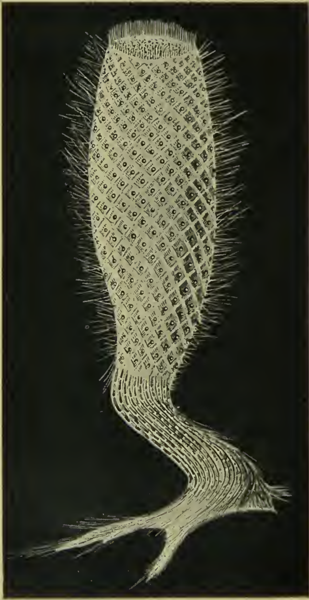
Fig. 3.— Euplectella suberea .
