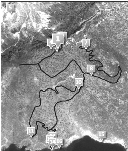
Εικόνα 39: Η διαδρομή Νικιά – Αυλάκι, όπου σημειώνονται οι θέσεις ενδιαφέροντος που αναφέρονται στο κείμενο.
