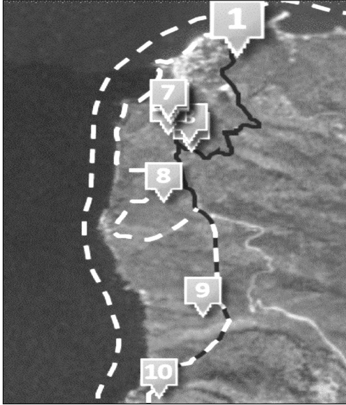
Εικόνα 41: Η διαδρομή Κάτερος, όπου σημειώνονται οι θέσεις ενδιαφέροντος που αναφέρονται στο κείμενο.
