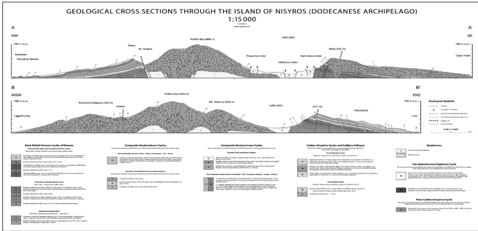
Εικόνα 19: Γεωλογικές τομές του ηφαιστείου της Νισύρου (Dietrich, 2018), όπου απεικονίζεται η σε βάθος κατανομή των γεωλογικών σχηματισμών καθώς και ένας αριθμός ρηγμάτων που διακόπτουν τη συνέχεια τους.
