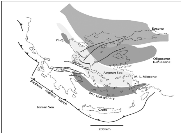
Εικόνα 16: Κατά προσέγγιση μετανάστευση του Ελληνικού Ηφαιστειακού Τόξου κατά τις περιόδους Ηώκαινο, Ολιγόκαινο – Κατώτερο Μειόκαινο, Μέσο - Ανώτερο Μειόκαινο, και Πλειόκαινο-Τεταρτογενές (Royden & Papanikolaou, 2011). Η Ελληνική τάφρος (Southern Hellenic Trench) συμβολίζεται με μια καφέ με τρίγωνα γραμμική και τα κανονικά και οριζόντιας μετατόπισης ενεργά ρήγματα στην ηπειρωτική Ελλάδα και στο Βόρειο Αιγαίο επισημαίνονται με μαύρες γραμμές με ή χωρίς δοντάκια.
