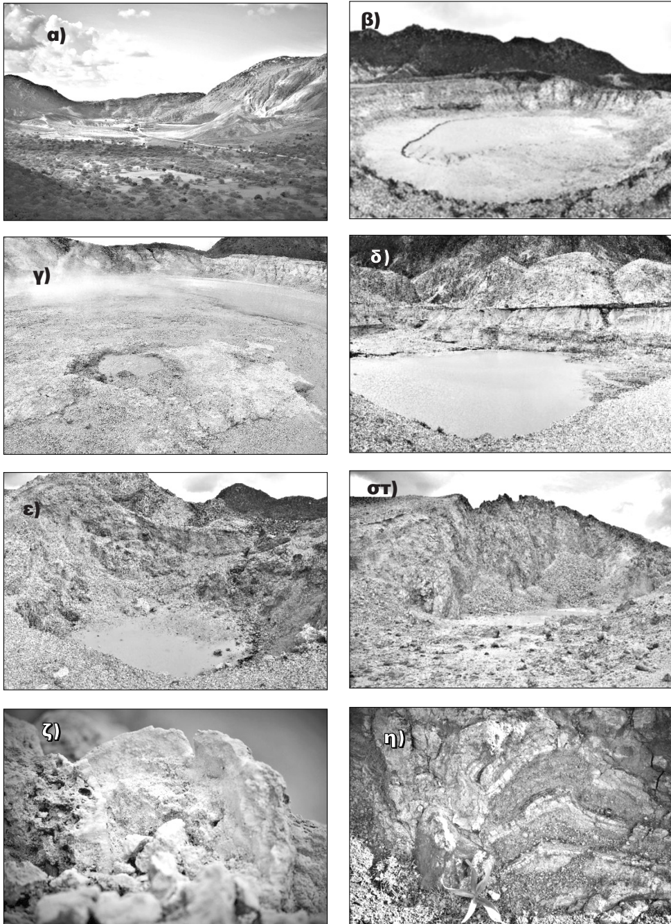
Εικόνα 29: Αντιπροσωπευτικές φωτογραφίες από τις θέσεις ενδιαφέροντος κατά μήκος της διαδρομής Καλδέρα-Λακκί: α) Θέα στους κρατήρες, β) Κρατήρας Στέφανος, γ) Λίμνη λάσπης, δ) Κρατήρας του Μεγάλου Πολυβώτη, ε) Κρατήρας του Μικρού Πολυβώτη, στ) Κρατήρας Λογοθέτης, ζ) Φουμαρόλες στον κρατήρα Στέφανος, η) Τόφφοι.
