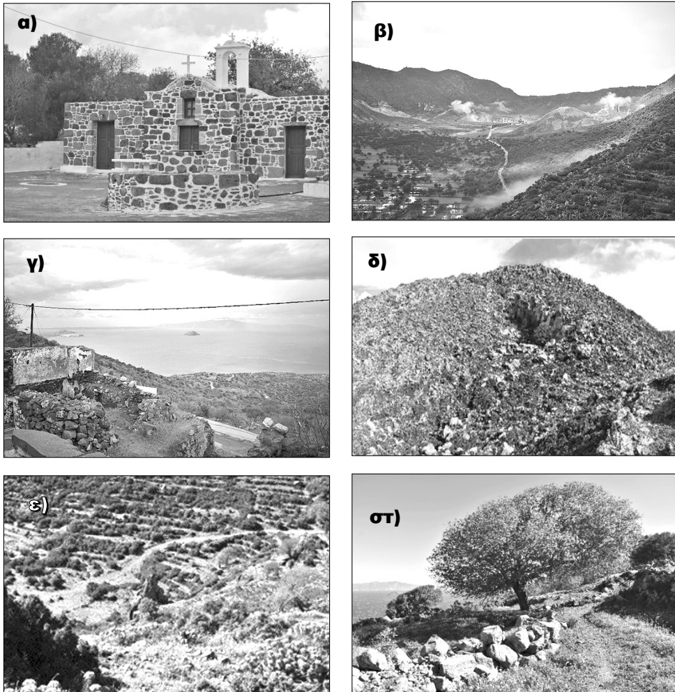
Εικόνα 46: Αντιπροσωπευτικές φωτογραφίες από τις θέσεις ενδιαφέροντος κατά μήκος της διαδρομής Ευαγγελίστρια - Εμπορείος: α) Μονή Ευαγγελίστριας, β) Θέα στους κρατήρες, γ) Θέα από τον Εμπορείο, δ) Λόφος Μποριάτικο, ε) Λαιμός λάβας, στ) Μονοπάτι.
