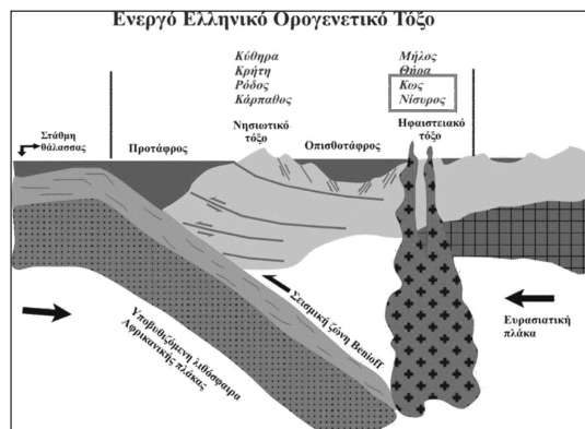
Εικόνα 13: Σχηματική Τομή του Ενεργού Ελληνικού Ορογενετικού Τόξου (Παπαϊωαννίδη, 2015).
