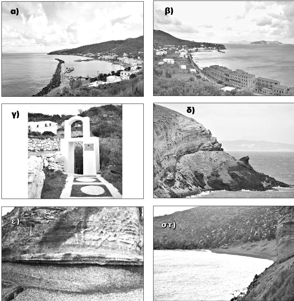
Εικόνα 44: Αντιπροσωπευτικές φωτογραφίες από τις θέσεις ενδιαφέροντος κατά μήκος της διαδρομής Πάλιοι – Λιές: α) Οικισμός Πάλιοι, β) Λουτρά Παντελίδη, γ) Θερμανή, δ) Βασαλτική ακολουθία, ε) Ροές δακτυλικής λάβας, στ) Παραλία Παχιά Άμμος.
