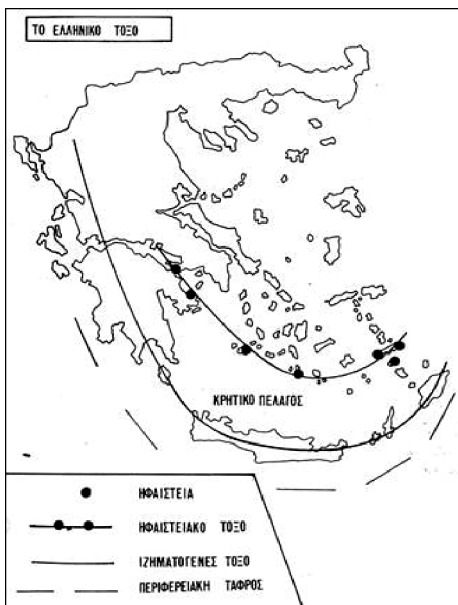
Το ελληνικό τόξο
