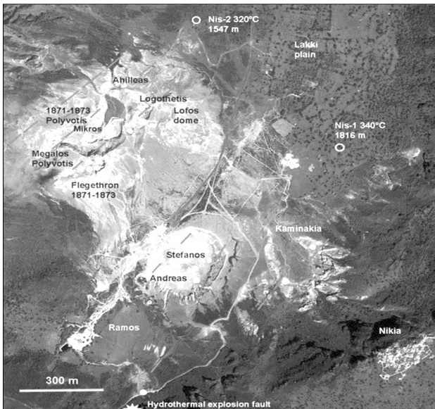
Εικόνα 30: Οι υδροθερμικοί κρατήρες της Νισύρου στο Λακκί, όπως διακρίνονται από τη δορυφορική εικόνα IKONOS (Dietrich, 2018).
