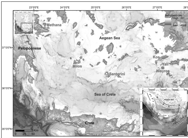
Εικόνα 14: Στιγμιότυπο οθόνης, στο οποίο απεικονίζονται τα ηφαιστεια που απαρτίζουν το ελληνικό ηφαιστειακό τόξο.
