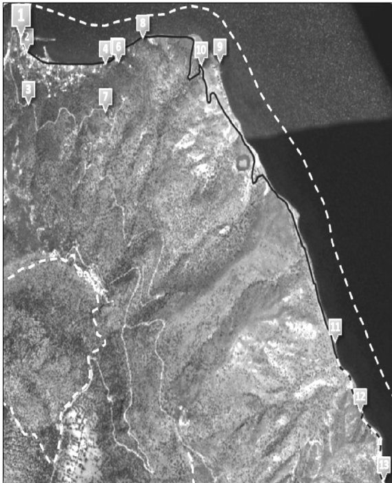
Εικόνα 43: Η διαδρομή Πάλαι-Λιές, όπου σημειώνονται οι θέσεις ενδιαφέροντος που αναφέρονται στο κείμενο.
