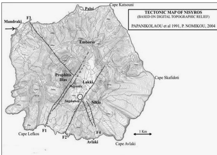
Εικόνα 20: Τεκτονικός χάρτης ρηξιγενών ζωνών της Νισύρου, F1-F4 τα κύρια ρήγματα (Παπανικολάου κ.α., 1989; 1991; Νομικού, 2004).
