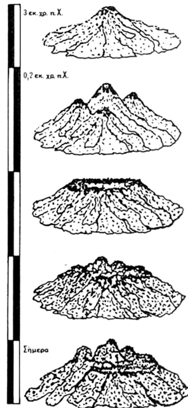
Ηφαιστειολογική εξέλιξη της Νισύρου
