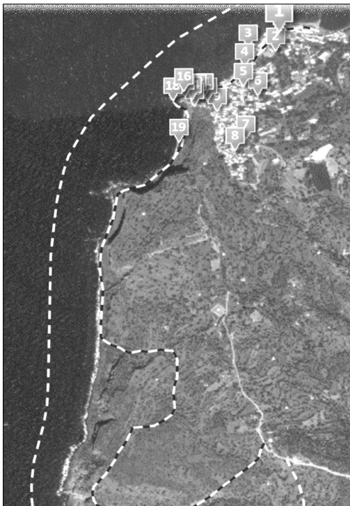
Εικόνα 35: Η διαδρομή Χοχλάκοι - Κανόνι, όπου σημειώνονται οι θέσεις ενδιαφέροντος που αναφέρονται στο κείμενο.
