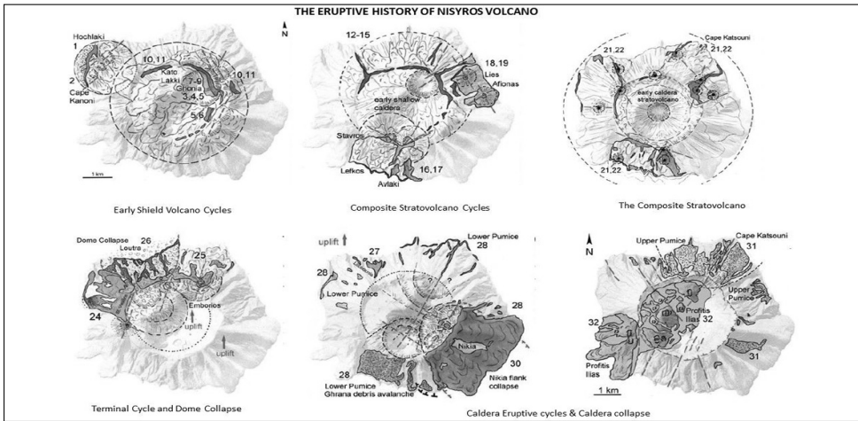
Εικόνα 22: Η εξέλιξη του ηφαιστείου της Νισύρου (από αριστερά προς τα δεξιά: αρχικές φάσεις ασπιδωτού ηφαιστείου, φάσεις σύνθετου στρωματοηφαιστείου, σύνθετο στρωματοηφαίστειο, τερματικός κύκλος και κατάρρευση καλδέρας, εκρηκτικές φάσεις καλδέρας και κατάρρευση καλδέρας). Οι αριθμοί αντιστοιχούν στους γεωλογικούς σχηματισμούς που αποτυπώνονται στον γεωλογικό χάρτη (Dietrich J.V., 2018).
