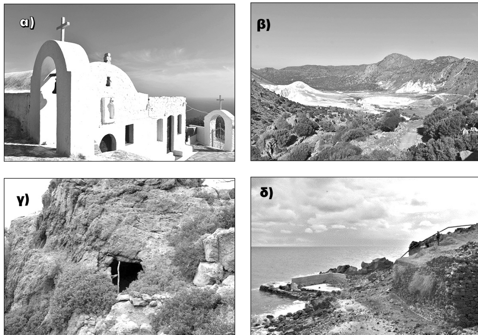
Εικόνα 34: Αντιπροσωπευτικές φωτογραφίες από τις θέσεις ενδιαφέροντος κατά μήκος της διαδρομής Άργος: α) Μοναστήρι Σταυρού, β) Θέα προς τους κρατήρες, γ) Δρακόσπηλιο, δ) Ερείπια εργοστασίου θείου στην Αγία Ειρήνη.
