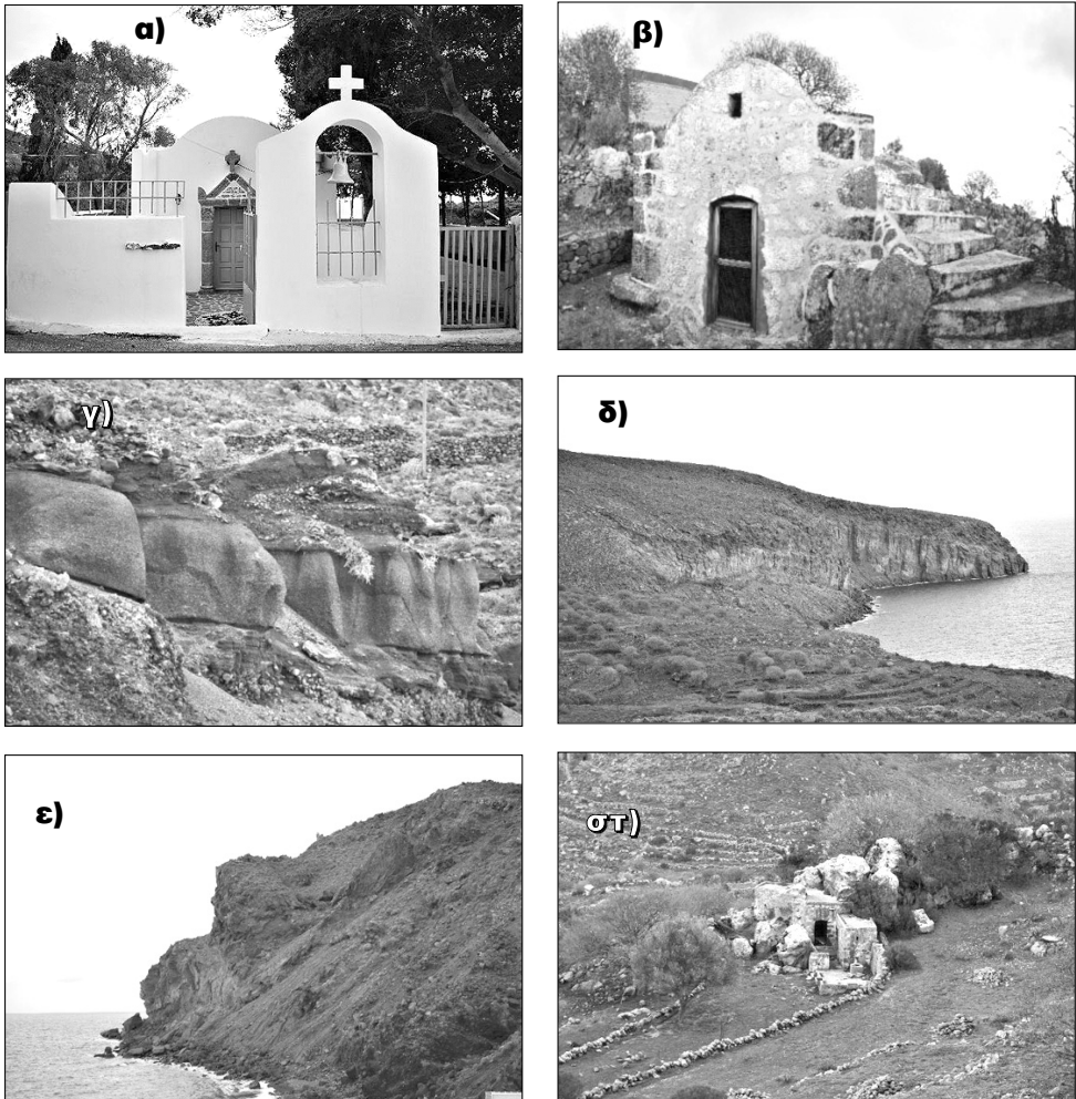
Εικόνα 40: Αντιπροσωπευτικές φωτογραφίες από τις θέσεις ενδιαφέροντος κατά μήκος της διαδρομής Νικιά – Αυλάκι: α) Εκκλησία Άγιος Παντελεήμονας, β) Αγία Τριάδα, γ) Σκωρίες, δ) Ρυολιθική πυροκλαστική ακολουθία, ε) Λάβες Ακρωτηρίου, στ) Αγροίγιες
