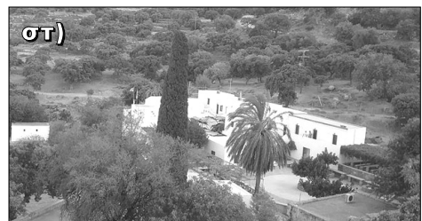
Εικόνα 38: Αντιπροσωπευτικές φωτογραφίες από τις θέσεις ενδιαφέροντος κατά μήκος της διαδρομής Νικιά – Φυλάκιο – Παρλέτια: α) Οικισμός Νικιά, β) Πλατεία Πόρτα (Νικιά), γ) Θέα στους κρατήρες, δ) Προφήτης Ηλίας Νικιών, ε) Παρλέτια, στ) Μονή Κυράς, ζ) Ρυολιθικές λάβες Νικιών.
