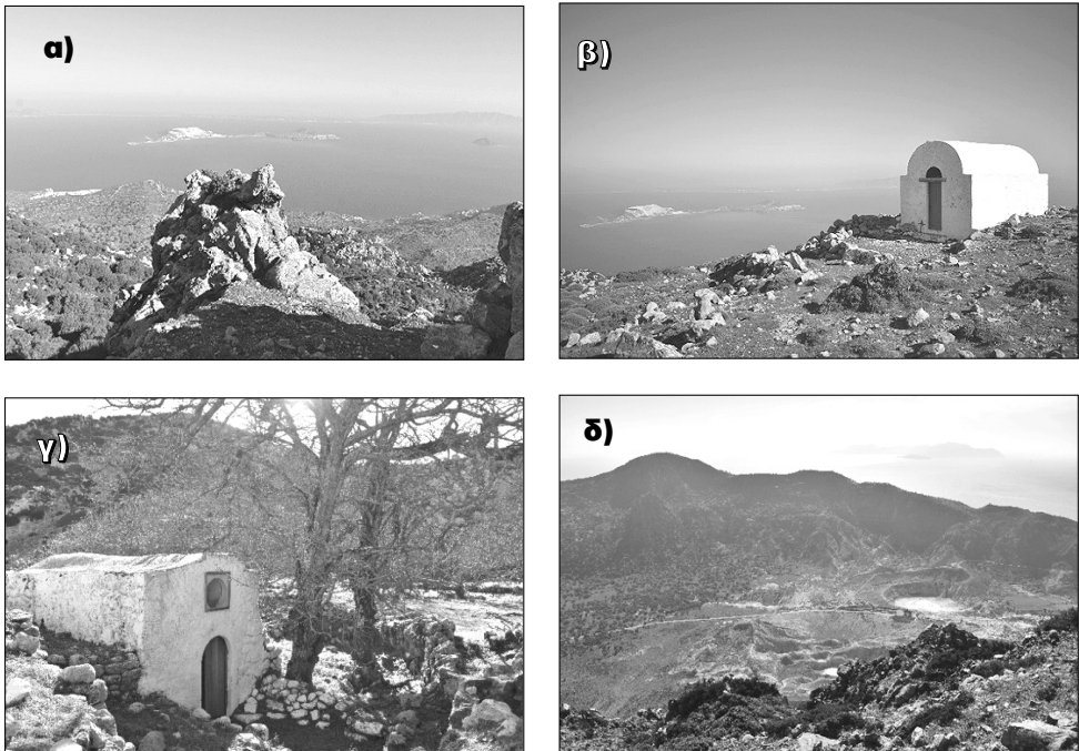
Εικόνα 32: Αντιπροσωπευτικές φωτογραφίες από τις θέσεις ενδιαφέροντος κατά μήκος της διαδρομής Διαβάτης – Νύφιος: α) Ρυοδακίτες, β) Προφήτης Ηλίας, γ) Παναγιά Διαβατινή, δ) Θέα προς κρατήρες από τον Προφήτη Ηλία.
