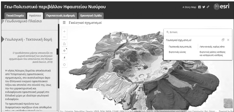
Εικόνα 18: Στιγμιότυπο οθόνης, το οποίο απεικονίζει την χωρική επιφανειακή κατανομή των γεωλογικών σχηματισμών που απαρτίζουν τη νήσο σύμφωνα με τον Dietrich (2018). Πρόκειται για έναν τρισδιάστατο διαδραστικό χάρτη, όπου ο χρήστης έχει τη δυνατότητα να τον περιστρέψει προκειμένου να περιηγηθεί σε αυτόν καθώς και να αντλήσει περισσότερες πληροφορίες επιλέγοντας έναν σχηματισμό.
