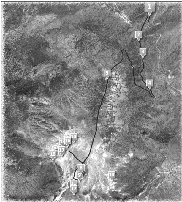
Εικόνα 28: Η διαδρομή Καλδέρα – Λακκί όπου σημειώνονται οι θέσεις ενδιαφέροντος που αναφέρονται στο κείμενο.
