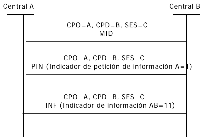
FIGURA 42.- Secuencia de los mensajes de información.
