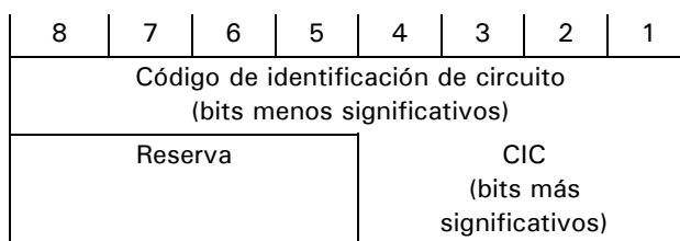
FIGURA 2.- Campo de identificación de circuito.
