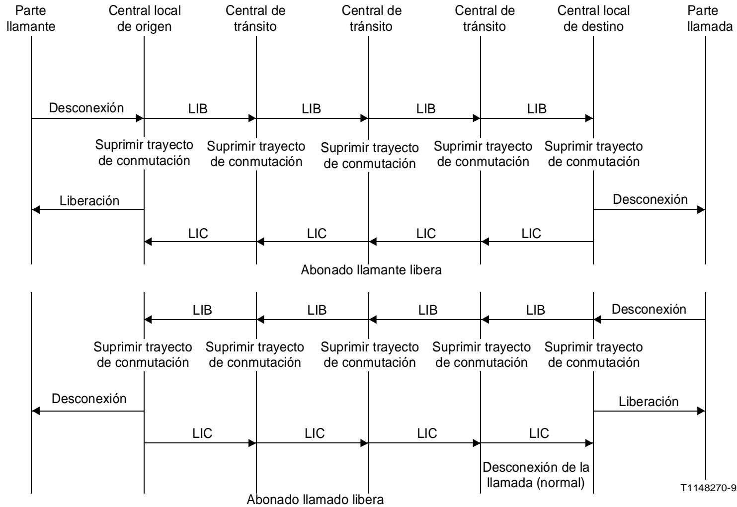
FIGURA 48.- Liberación de llamada normal.
