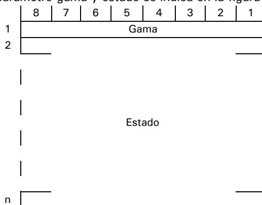
FIGURA 24.- Campo del parámetro gama y estado.
