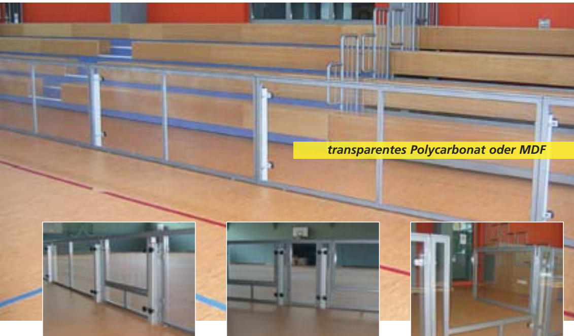
Bande mit Ausleger
