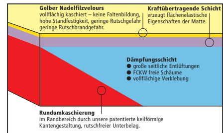
Schnitt durch FIG-Niedersprungmatten-Sandwich
