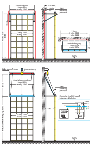
Elektrisch hochziehbare Gitterleiter in Betriebstellung
