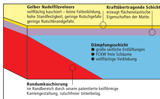
Schnitt durch FIG-Niedersprungmatten-Sandwich
