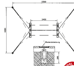
Distanzhalterung
