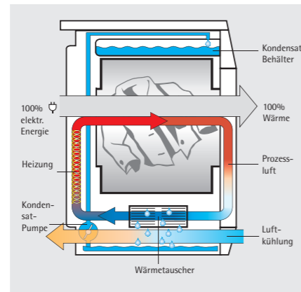
Schema: Kondensations-Trockner
