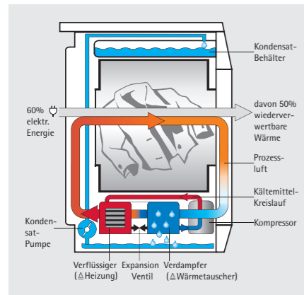
Schema: Wärmepumpen-Trockner
