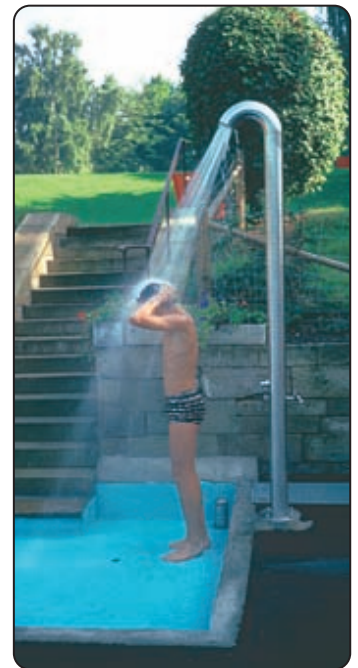
Einfach-Standbrause V2A-Edelstahl-Rundrohr Ø 108 mm, geschliffen, innenliegender MS-verchromter Brausekopf einschließlich einstellbarem Selbstschlussventil 1/2", Befestigung mittels Bodenflansch, Wasserzuleitung 3/4". 9377 Preis auf Anfrage
