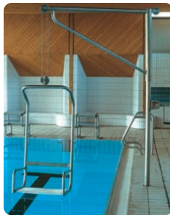
Versehrten-Lift Handwindenbetrieb, schwenkbar in Bodenhülse gelagert, herausnehmbar. Komplette Edelstahlausführung. 9359 Preis auf Anfrage
