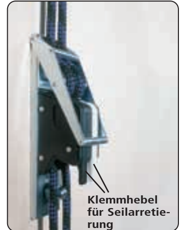
Gebrauchsstellung - die Sicherheitseinrichtung ist aktiv, unbeabsichtigtes Öffnen der Klemmhebel für Seilarretierung nicht mehr möglich.
