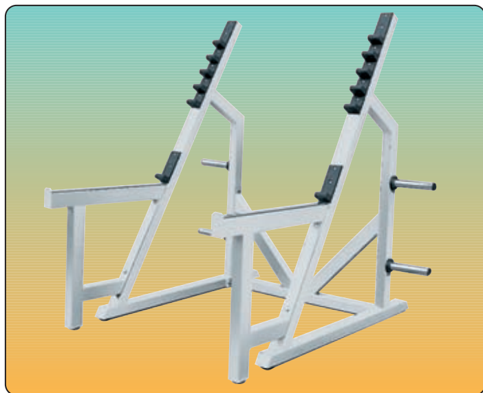
GRIZZLY POWER® Kniebeugeständer mit Sicherheitsablage aus Stahlprofilrahmen-Elementen die miteinander verschraubt werden. Maße: ca. 178x170x173 cm, Gewicht: ca. 90 kg.
