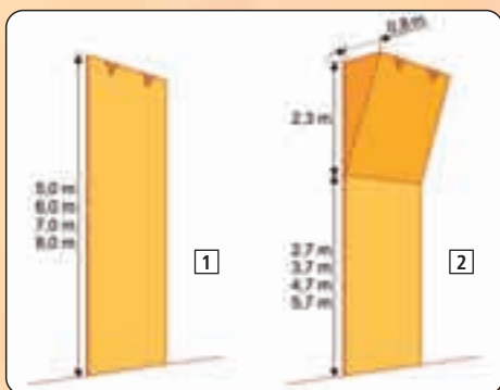
1 Modul MTM-01
