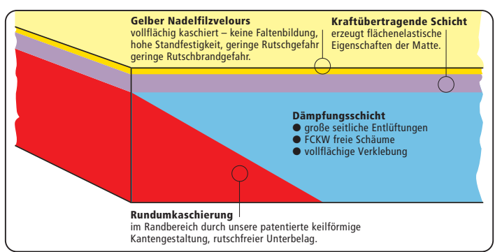
Schnitt durch BENZ® FIG-Niedersprungmatten-Sandwich
