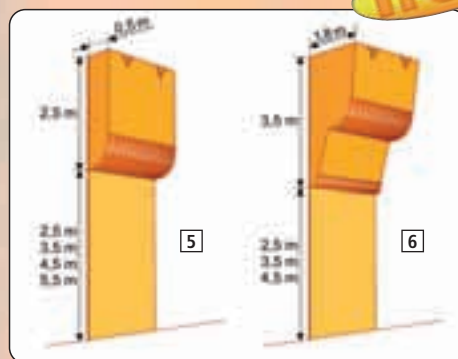
5 Modul MTM-05
