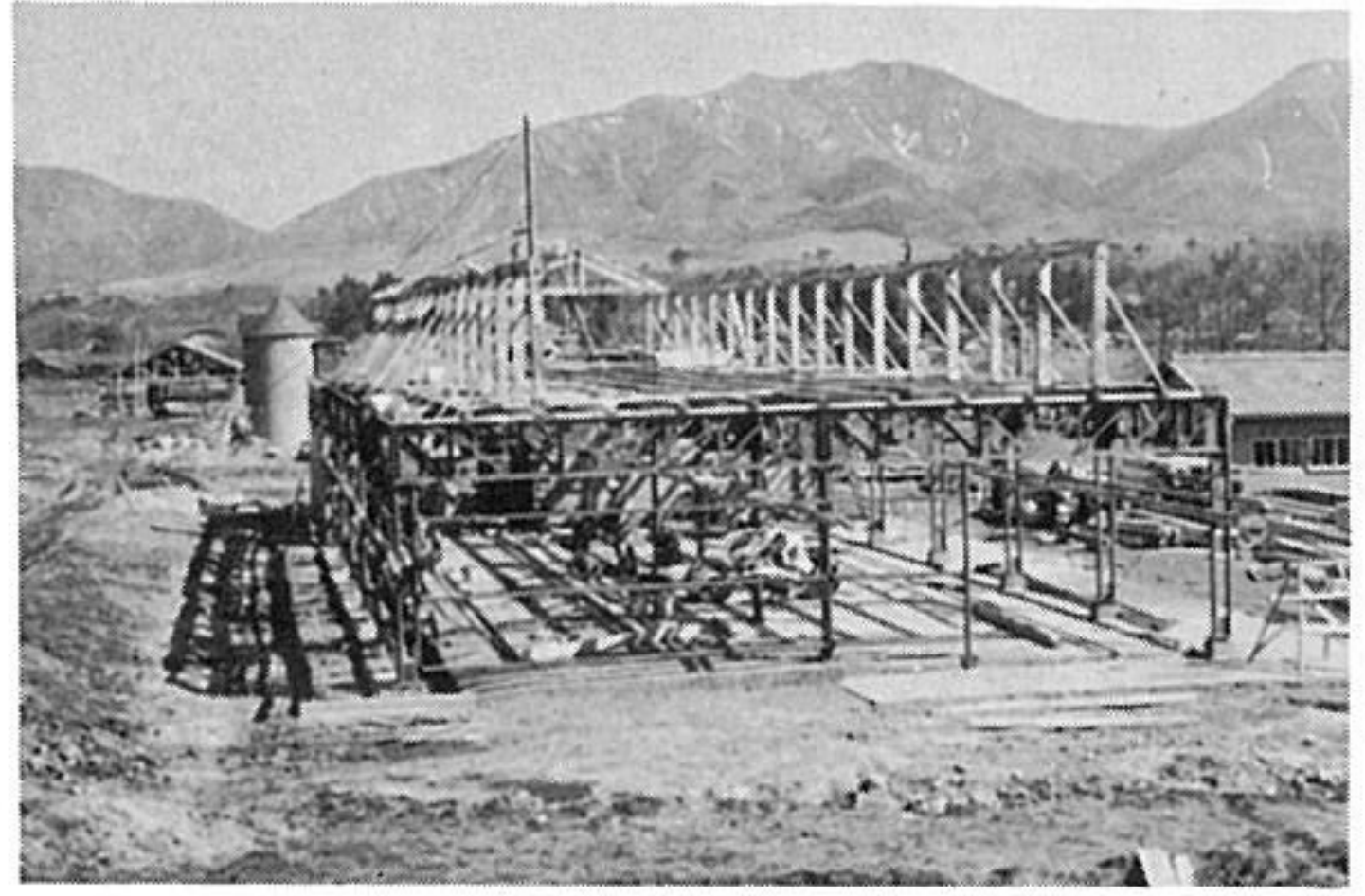
第1 牧場牛舎の建設
