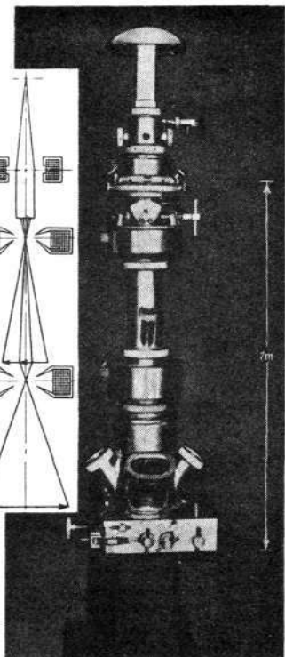
Elektronmikroskop.
