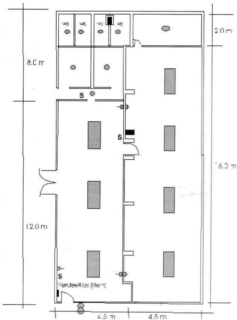
Grondplan van Hall of Fame
