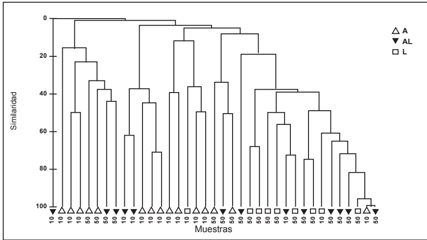
Figura 4. Clasificación basada en el índice de Bray Curtis por profundidad (50 y 10 m) y tipo de sedimento de los arrastres realizados en la plataforma continental de La Guajira. A: arena, AL: arena lodosa, L: lodo.
