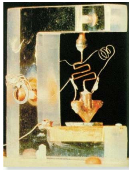
Figura 10. Primer transistor (6).
