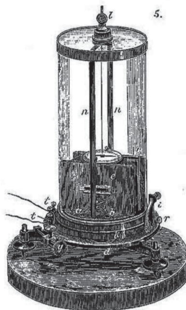
Figura 15. Galvanómetro de du Bois-Reymond; sólo detectan el paso de la corriente eléctrica pero no dan indicación de su magnitud ni del valor de la fuerza que la impulsa (10).
