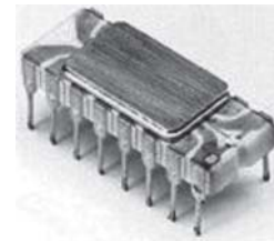
Figura 12. Intel 4004. Primer microprocesador (1971) (en un circuito integrado todo el procesador de una computadora), desarrollado por los ingenieros Ted Hoff y Federico Faggin en Intel; fue el 4004, de 4 bits y 275 transistores (6).
