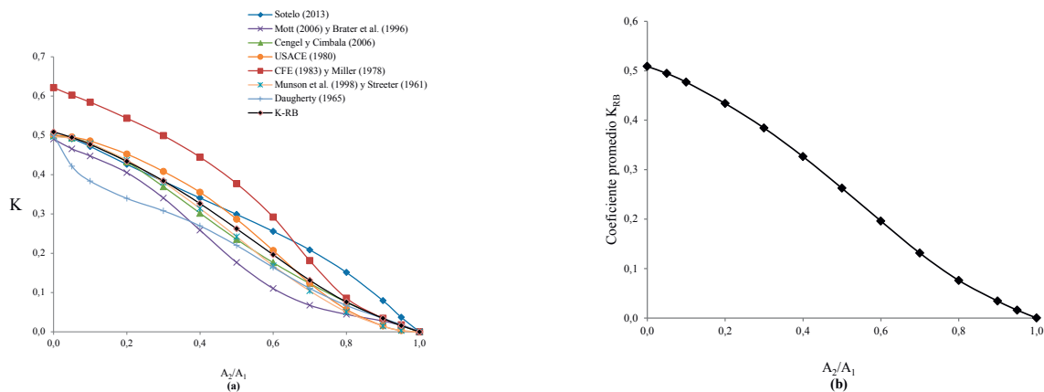
Figura 3. (a) Curvas del coeficiente K para una reducción brusca del diámetro, de acuerdo a la variación de la relación del área menor respecto a la mayor A_2/A_1 . La curva de K-RB es la representativa de los valores promedio. (b) Curva de ajuste a los valores del coeficiente K_{RB} , de acuerdo a la variación de la relación del área menor respecto a la mayor A_2/A_1 . Fuente: Elaboración propia, 2015.
