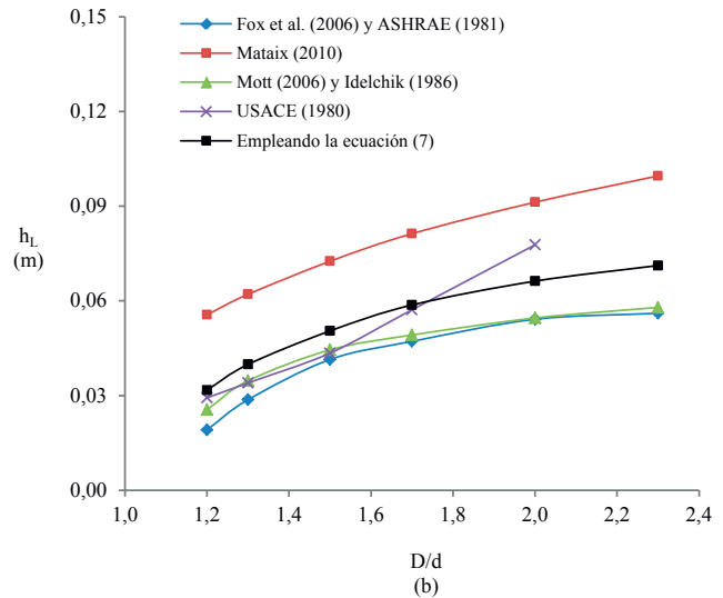
Figura 6. Comportamiento de las pérdidas de energía que generan dispositivos de reducción gradual del diámetro, estimadas bajo los lineamientos de la literatura que se indican y mediante la ecuación (7) propuesta en el presente trabajo, cuando el flujo desarrolla una velocidad promedio aguas abajo del dispositivo de: a) 1,5 m/s, b) 2,5 m/s. Fuente: Elaboración propia, 2015.
