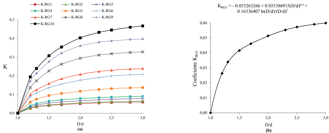
Figura 4. (a) Curvas de valores promedio del coeficiente K_{RG} de acuerdo a la relación del diámetro mayor con respecto al menor del dispositivo ( D/d ). (b) Curva de ajuste para los valores promedio del coeficiente K_{RG1} en función a la relación del diámetro mayor con respecto al menor del dispositivo ( D/d ). Fuente: Elaboración propia, 2015.
