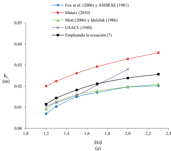
Figura 6. Comportamiento de las pérdidas de energía que generan dispositivos de reducción gradual del diámetro, estimadas bajo los lineamientos de la literatura que se indican y mediante la ecuación (7) propuesta en el presente trabajo, cuando el flujo desarrolla una velocidad promedio aguas abajo del dispositivo de: a) 1,5 m/s, b) 2,5 m/s. Fuente: Elaboración propia, 2015.
