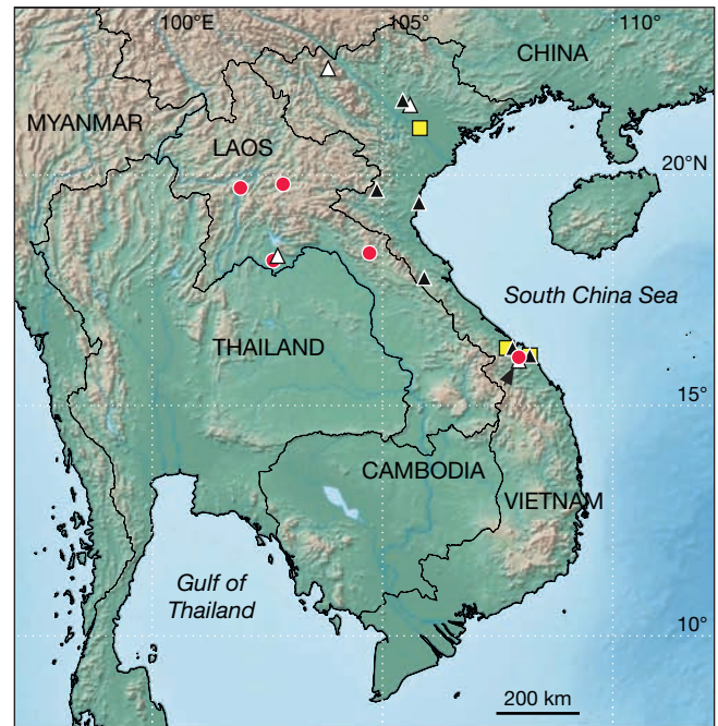
FIG. 42. — Distribution of Syzygium tonkinense (Gagnep.) Merr. & L.M.Perry (■), Syzygium tsoongii (Merr.) Merr. & L.M.Perry (▲), Syzygium vestitum Merr. & L.M.Perry (△) and Syzygium zimmermannii (Warb. ex Craib) Merr. & L.M.Perry (●) in Indochina.
