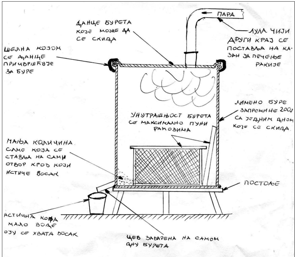
Казан за ракију као шпонионик за восак (цртеж Мирослава Васиљевића)
