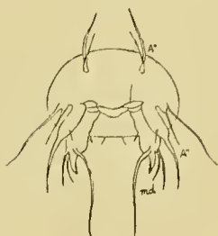
Fig. 21. - Primo stadio naupliiforme di Phyllothalestris mysis , × 126 circa.
