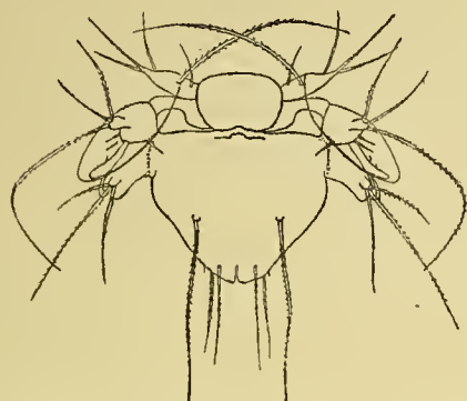
Fig. 18 - Terzo stadio naupliiforme di Altheutha interrupta ,? x 147 circa.
