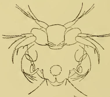
Fig. 12. - Terzo stadio naupliiforme di Harpacticus uniremis , \times 147 circa.
