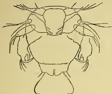
Fig. 13. - Altro Metanauplius di Harpacticus uniremis , (stadio incerto) lungo mm. 0,22, \times 147 .
