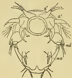
Fig. 8. - Terza forma metanaupliiforme (quarto nauplio) di Psamathe longicauda , × 101 circa.
