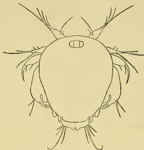
Fig. 14 - Quinto stadio naupliforme di Harpacticus uniremis (larva vista dal lato dorsale), \times 141 circa.
