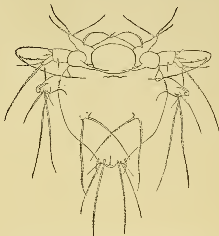
Fig. 19. - Quarto stadio naupliiforme di Altheutha interrupta ,? x 150 circa.
