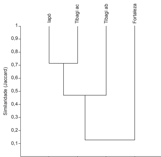
Figura 4. Dendrograma de similaridade (Jaccard) entre os trechos de rios da bacia do rio Tibagi, no período de maio de 2001 a abril de 2002.
