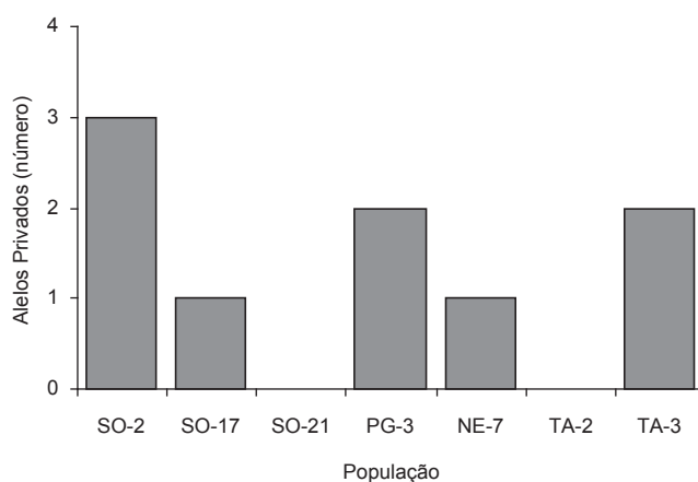
Figura 3. Frequência de alelos privados em sete populações de Oryza glumaepatula .
