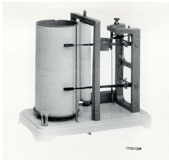
Termoigrografo meccanico
