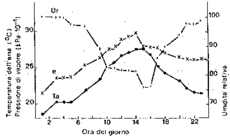
Fig. 4.6 – Andamento giornaliero tipico della temperatura dell'aria (•), pressione di vapore (x), umidità relativa (+), sopra una coltura di soia (da Rosenberg ed altri).
