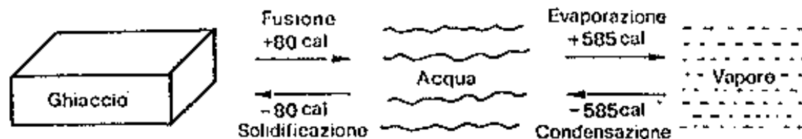
Fig. 4.1 – Calorie assorbite (+) e cedute (–) da un grammo di acqua nei cambiamenti di stato. Il valore dato per l' evaporazione e la condensazione è solo indicativo poiché esso varia con la temperatura approssimativamente con una legge del tipo:
