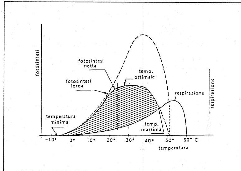
Figura 8.3. Relazioni tra temperatura, fotosintesi e respirazione. La fotosintesi netta (area tratteggiata) è data dalla somma algebrica tra fotosintesi lorda e respirazione.
