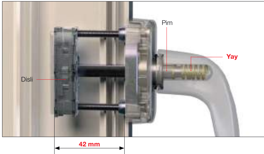
VarioFit® pencere kolu, pim uzunluğu 42 mm
