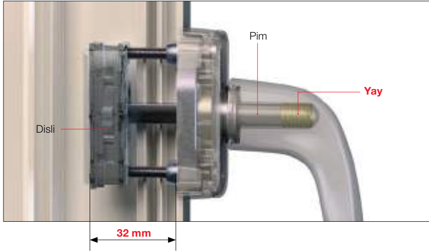
VarioFit® pencere kolu, pim uzunluğu 32 mm
