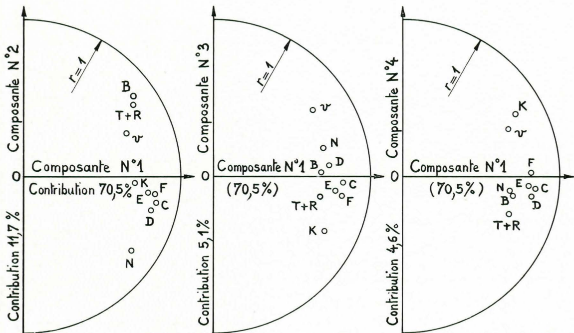
FIG. 2. — Représentation des caractères initiaux par leurs coefficients de corrélation avec les premières composantes principales (Analyse I).
