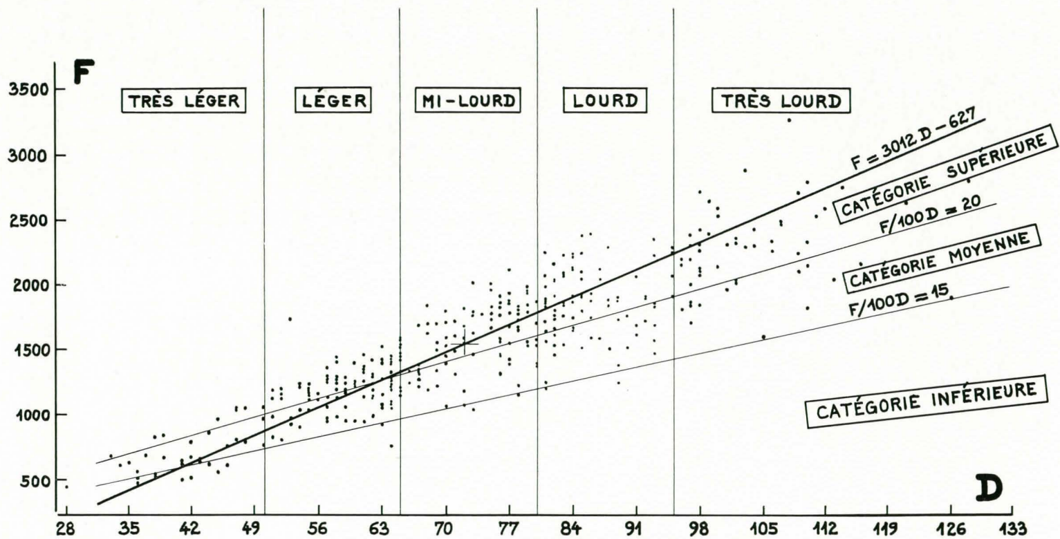
FIG. 20 — Le nuage dans le plan D-F.
