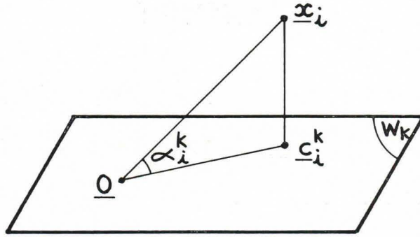
FIG. 23. — Projection d'un individu dans un sous-espace vectoriel.
