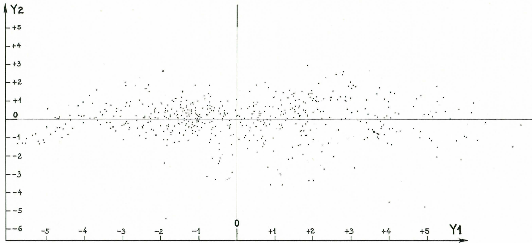
FIG. 4. — Le nuage des 565 points dans le plan des deux premières composantes principales.
