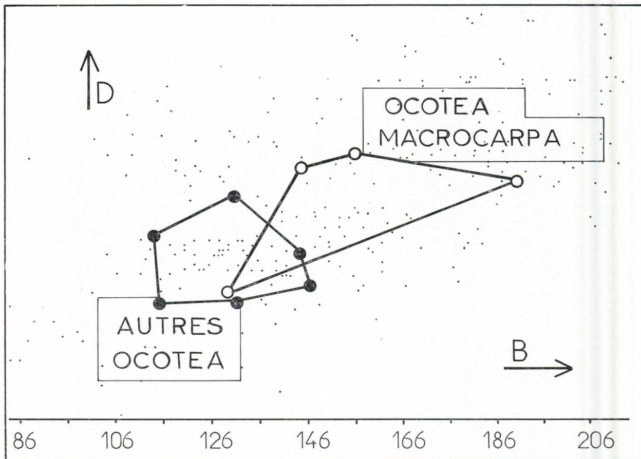
FIG. 21. — Comparaison Ocotea macrocarpa — autres Ocotea dans le plan B-D.
