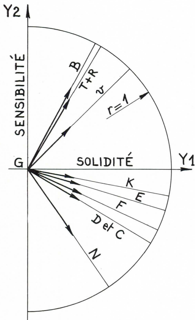
FIG. 5. — Projections dans le premier plan principal des vecteurs unitaires de l'ancien système de référence (caractères initiaux).
