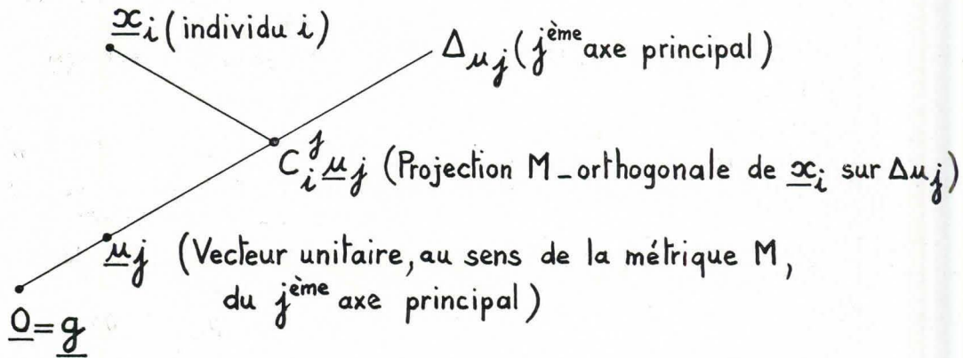
FIG. 24. — Projection d'un individu sur un axe principal.
