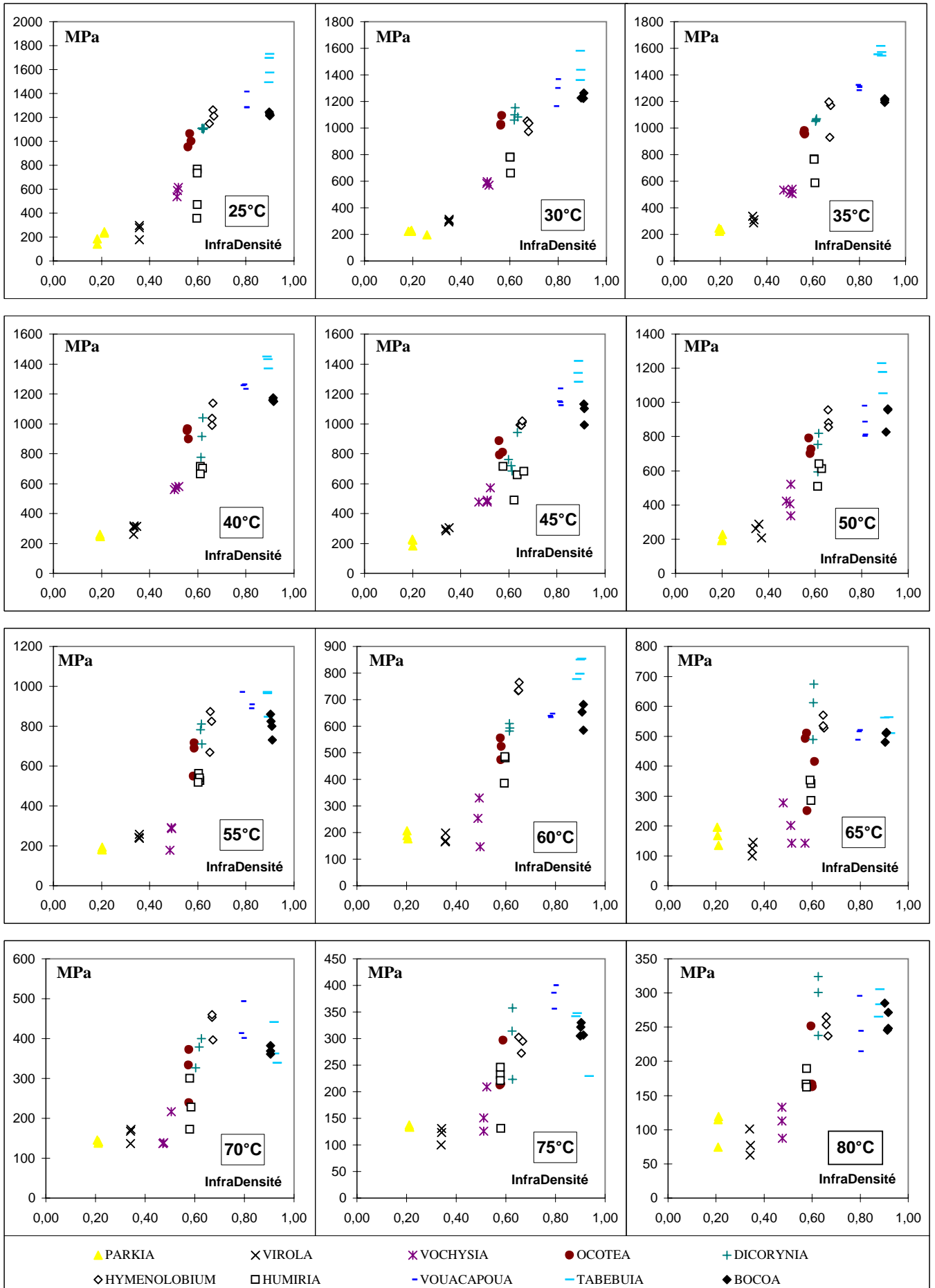
Evolution du module équivalent E_{re} (en MPa) de la courbe decompression radiale en fonction de l'infra-densité des dix espèces aux différentes températures d'essai.
