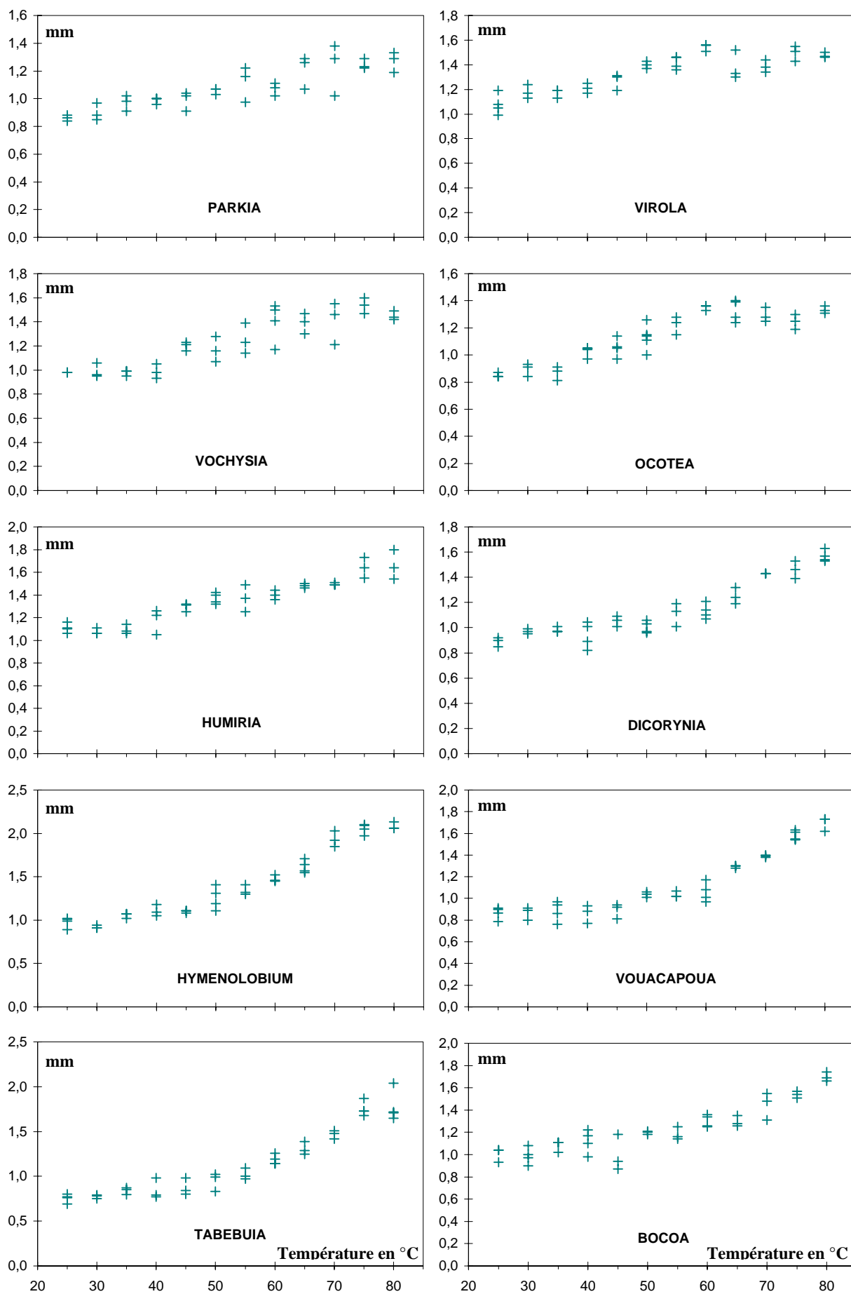
Evolution de la flèche à la rupture : f_{r,I} (en mm) de la courbe deténacité en fonction de la température pour chacune des dix espèces
