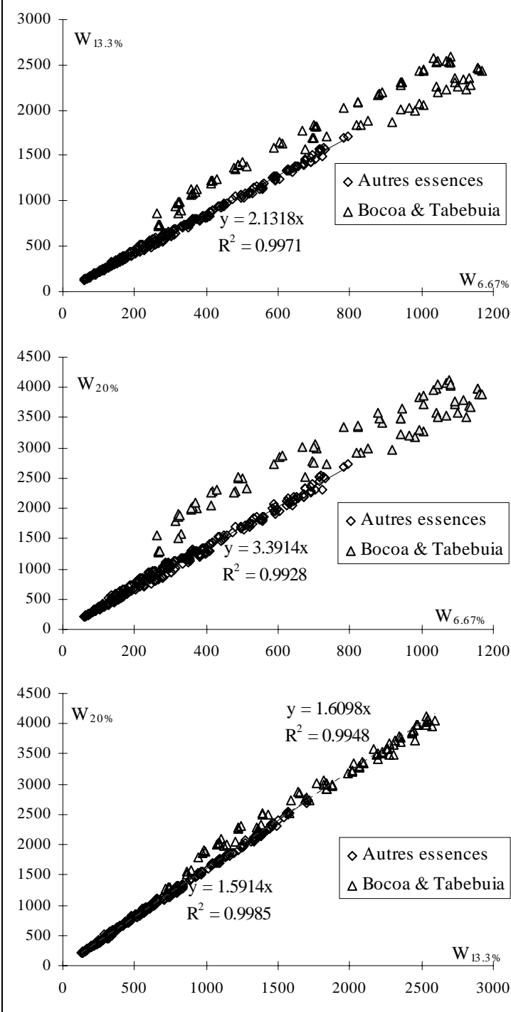
Figure IV - -7 Relation entre les différents W_{\epsilon\%}
