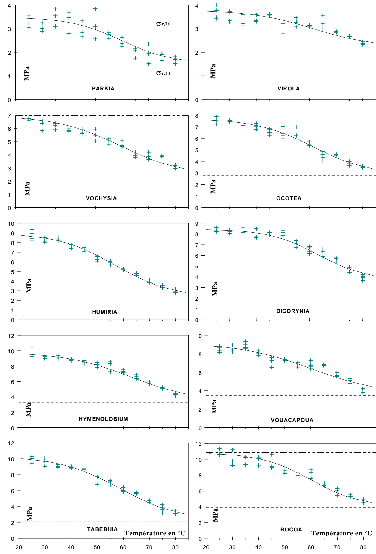
Figure IV - -43 Evolution de \sigma_{r,i} en fonction de la température pour les dix essences, les asymptotes en zéro et à l'infini sont représentées en pointillés.
