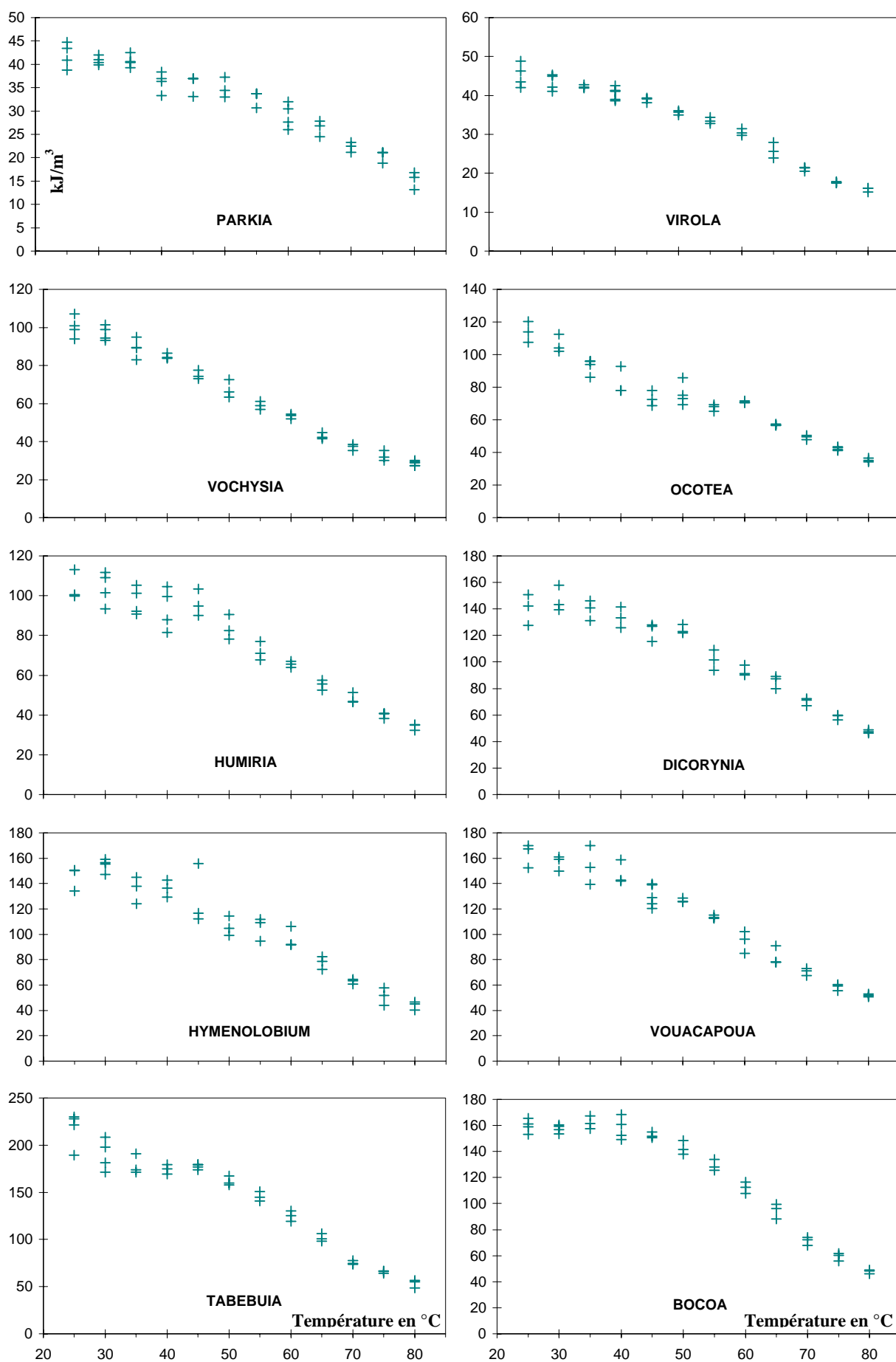
Evolution de l'énergie decisaillement pour un angle de cisaillement de 2.3° :W 2.3° (en kJ/m 3 ) en fonction de la température pour chacune des dix espèces.
