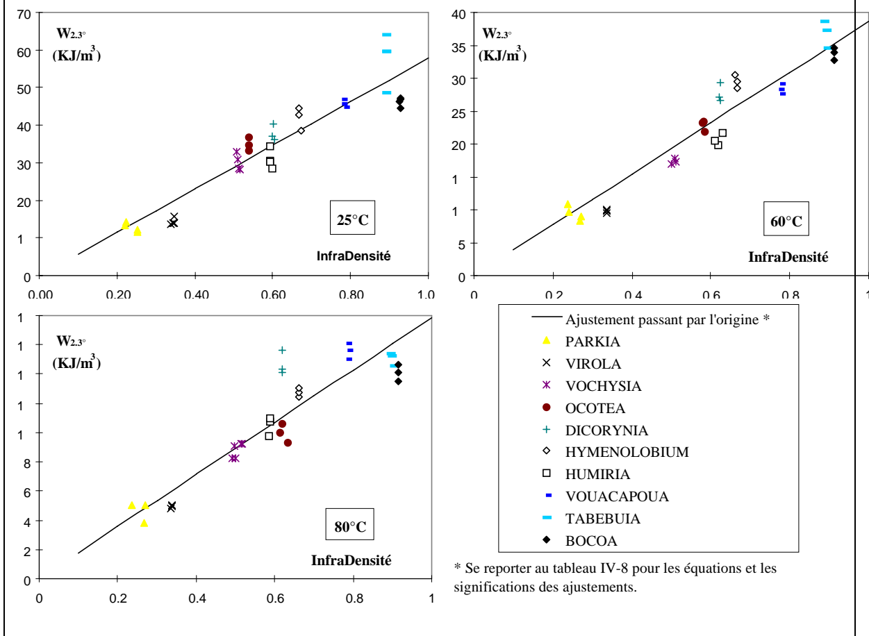
Figure IV - -30 Exemple d'ajustements de W_{2,3} en fonction de l'infradensité pour trois températures différentes
