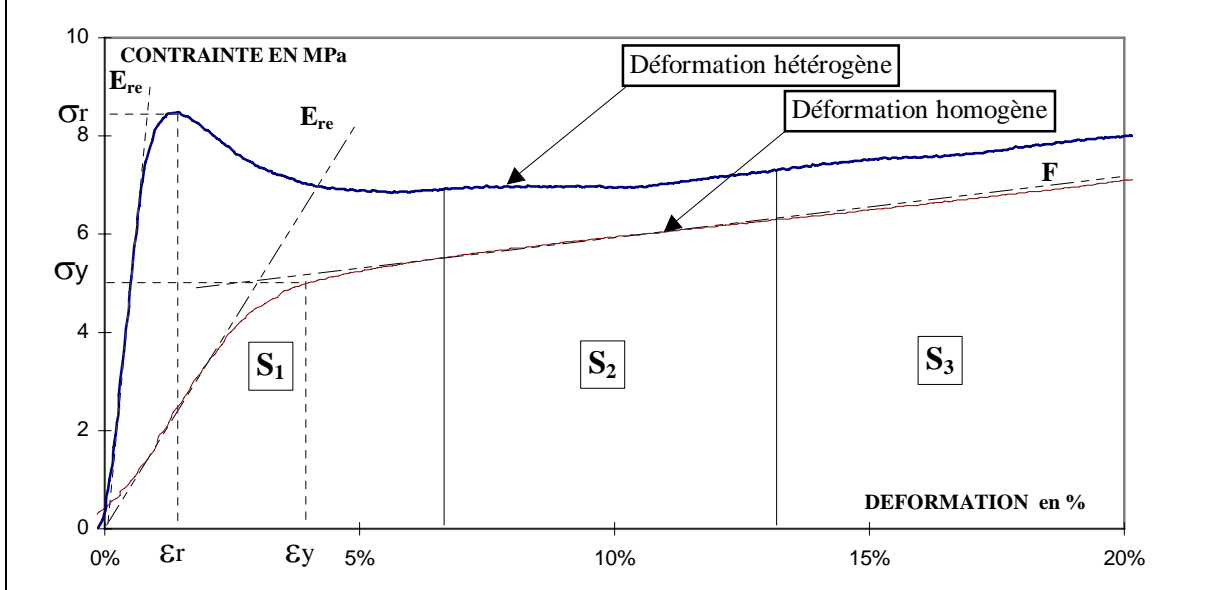
Figure III - -16 Paramètres descripteurs des courbes de compression
