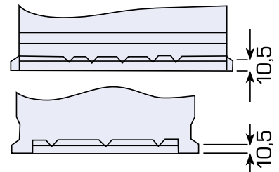
Bodenleiste B13
