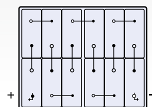
Schaltung 24V DIN C
