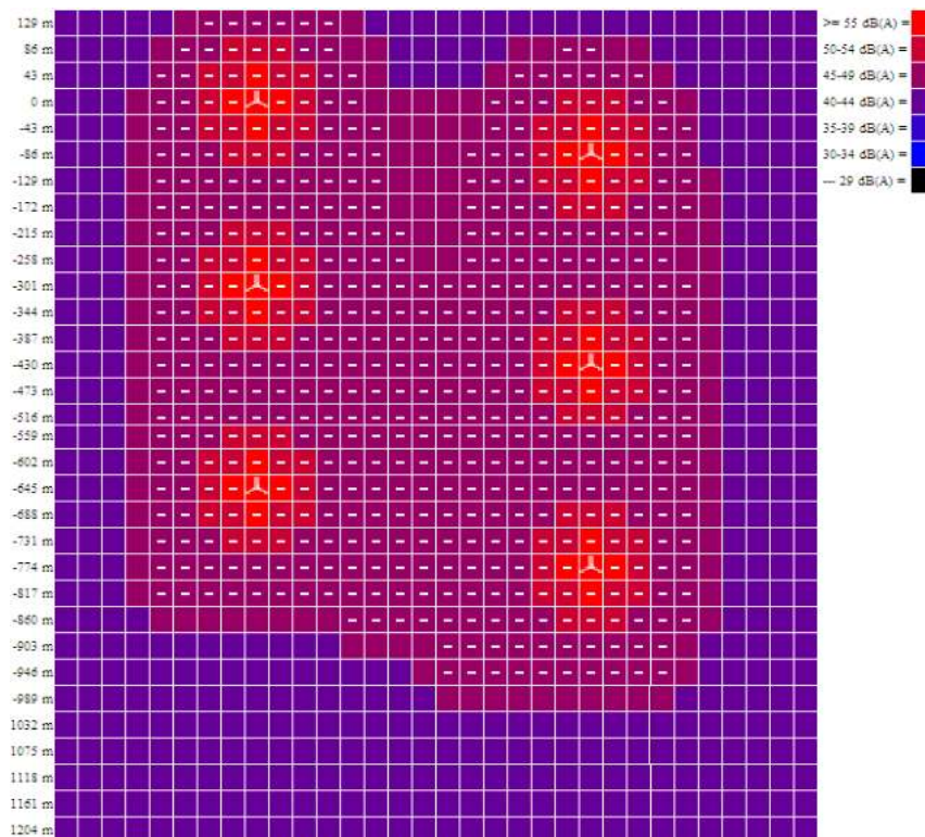
Niveles de sonido alrededor de aerogeneradores
