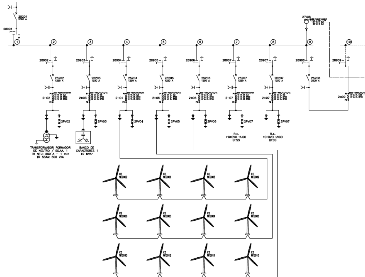
Figura 9. Esquema Unifilar Semibarra I: La Flecha Fuente: Aluar/Goldwind
