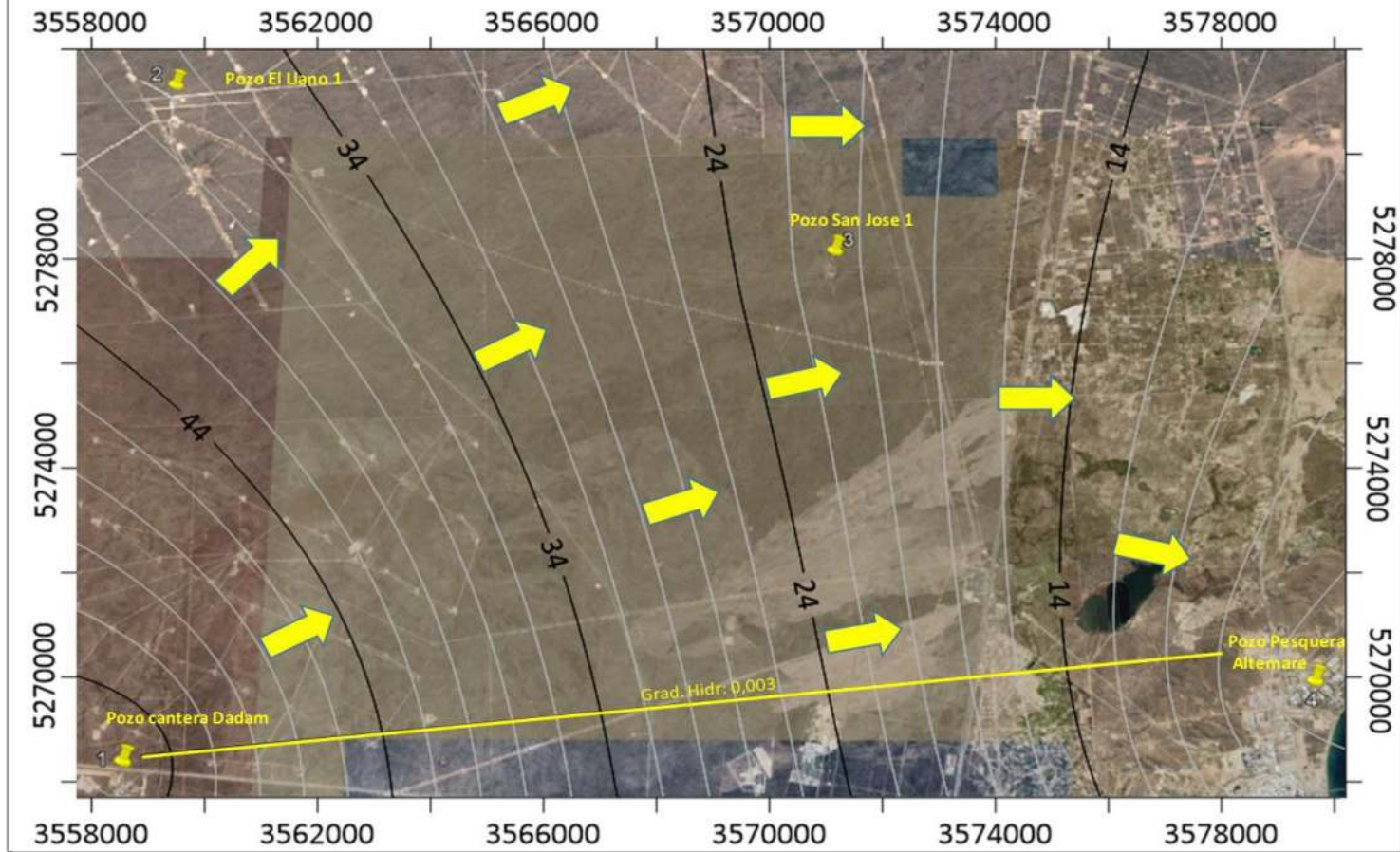
Figura 12. Plano isopiezas del Parque Eólico Aluar - Curvas isopiezas expresadas en m.s.n.m Fuente: Clasto SRL
