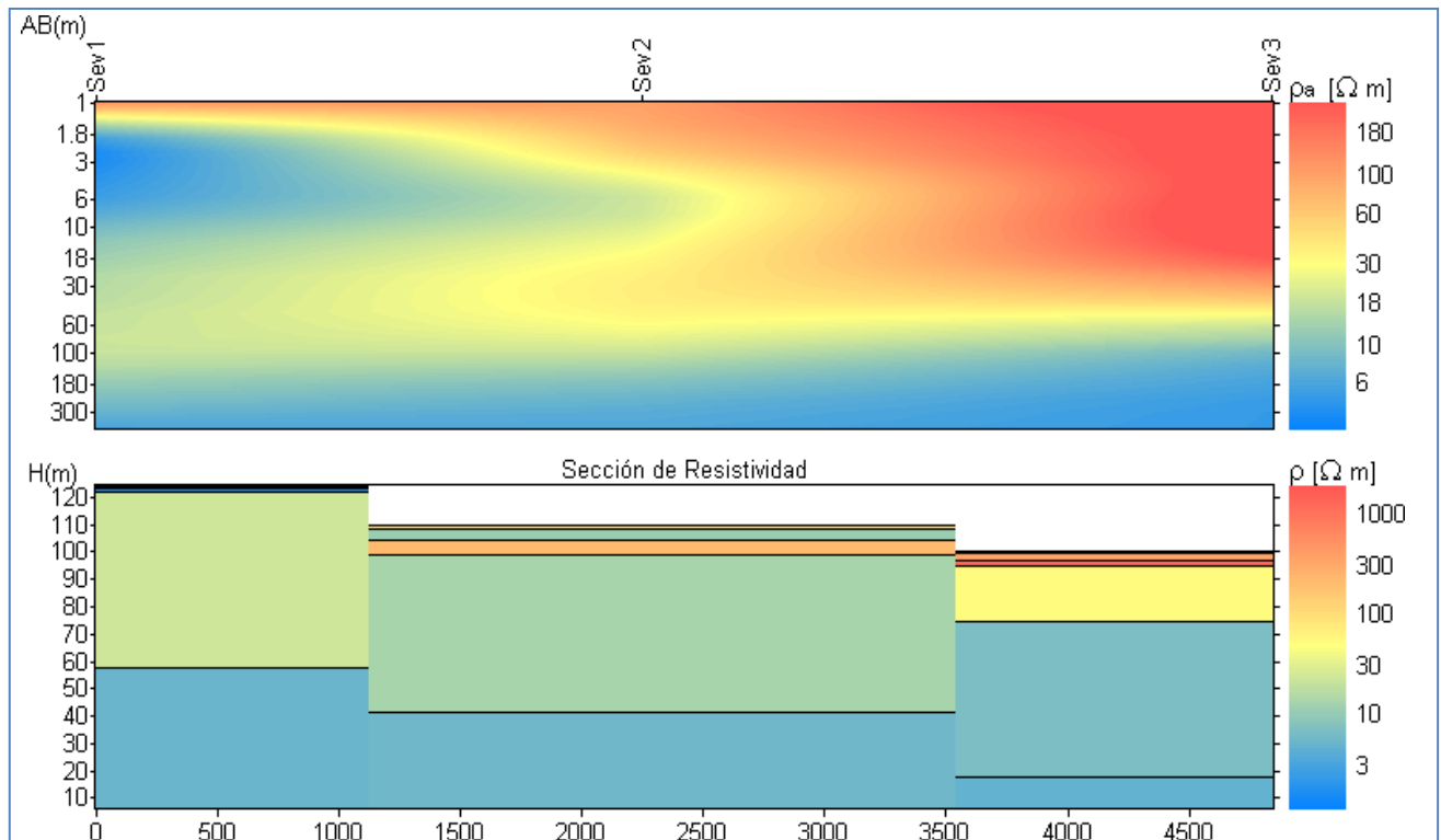
Figura 7. Sección resistiva SEV 1, 2 y 3
