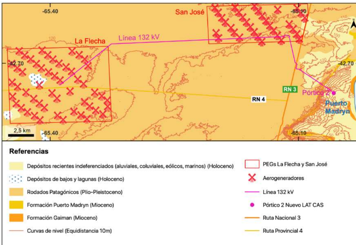
Figura 2. Geología general y curvas de nivel en las áreas destinadas al desarrollo del Parque Eólico ALUAR – Etapas V y VI – (extraído y simplificado de Haller et al., 2005).
