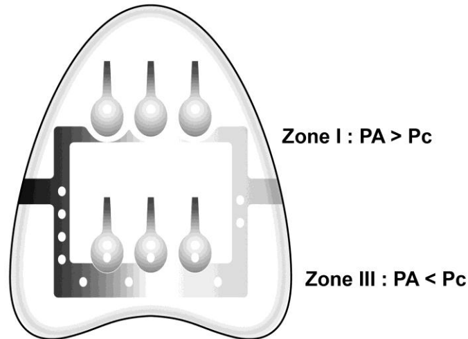
Figure 8.2 Zones de West simplifiées. Les zones I et III seulement sont représentées. (PA: pression alvéolaire; Pc: pression capillaire; les points blancs correspondent aux molécules de CO 2 dans la circulation sanguine).
