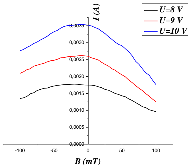
3-rasm. Kuchlanishni o'zgarmas qiymatlari uchun tok kuchini magnit maydon induksiya vektoriga bog'liqligi
