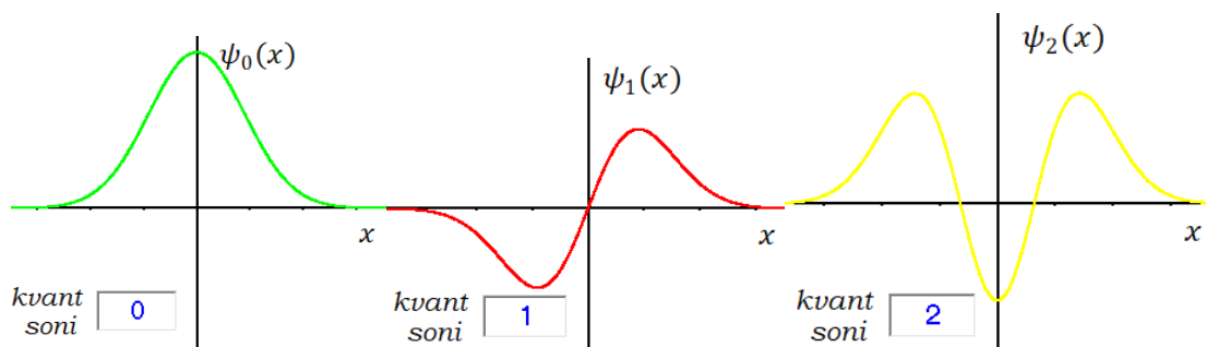
3-rasm. Kvant sonining turli qiymatlarida uchun to'liqin funksiyasining grafigi.
