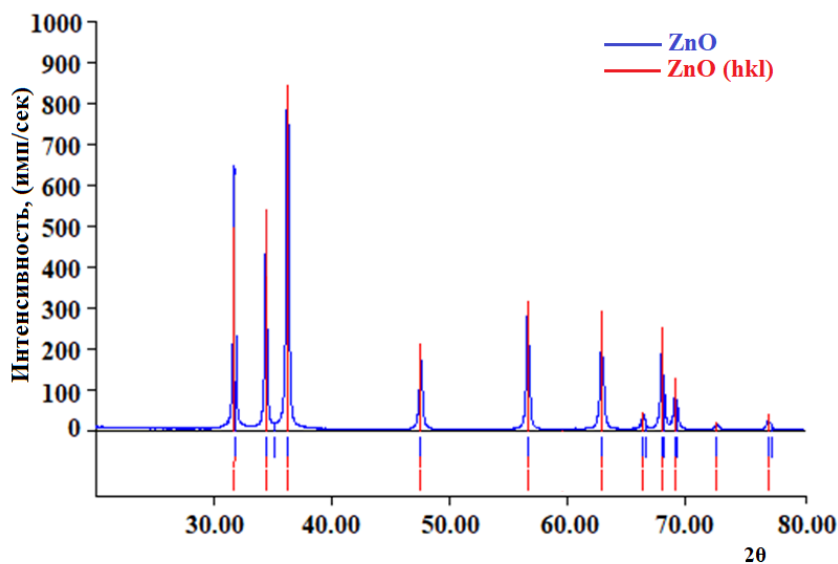
Рис.2.б) Спектральная зависимость ZnO после отжига при температуре 800°C, а также фазовый состав данного образца и индексы Миллера, определенные методом с помощью метода Search Match! с Ритвельдовским уточнением.
