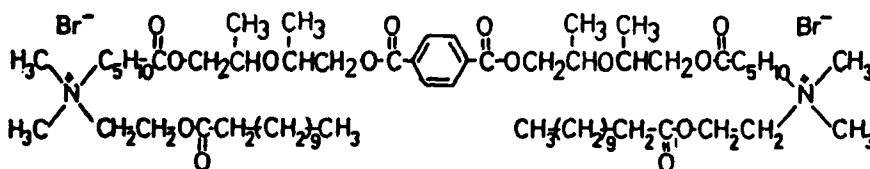
SCHEME 5. \text{diN}^+\text{-H} .
