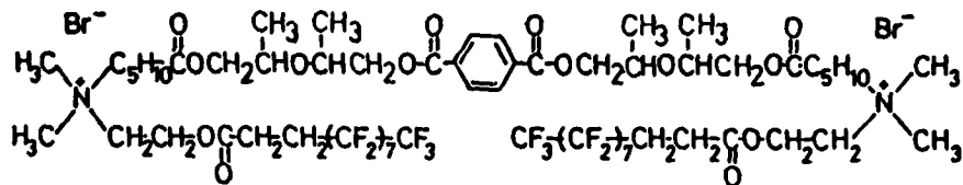
SCHEME 6. diN + -F.
