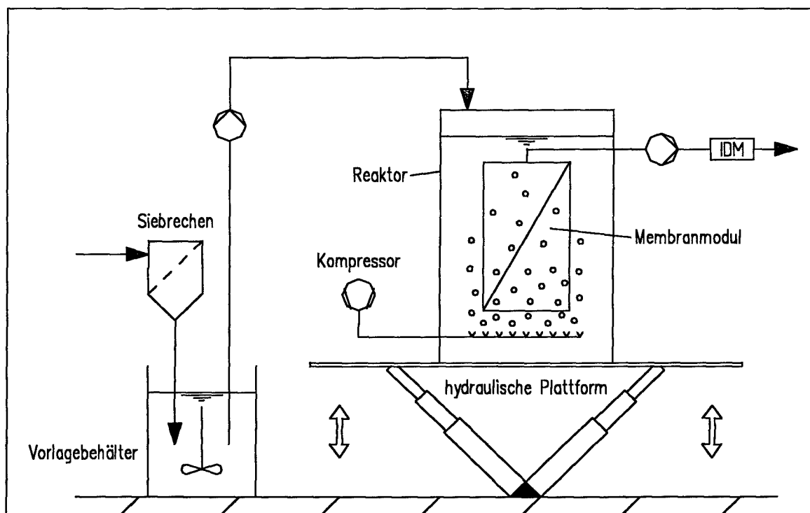
Bild 3: Aufbau der halbtechnischen Membranbioreaktoranlage -7-
