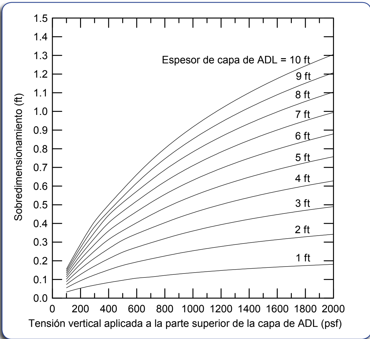
FIGURA D-2. Diagrama de diseño del sobredimensionamiento para ADL Tipo B
