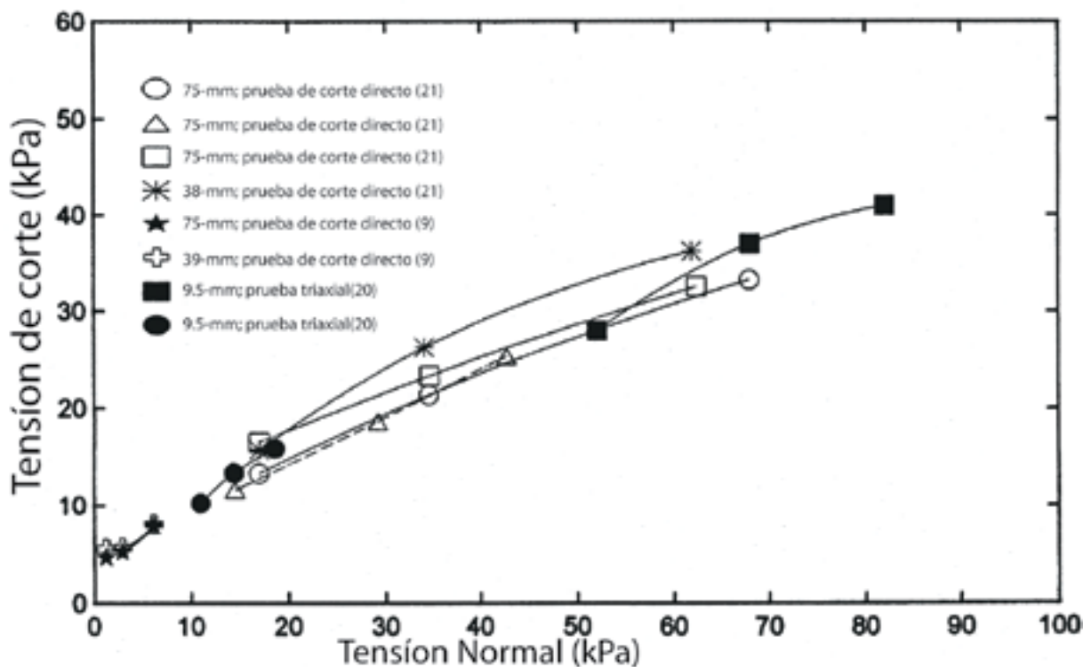
Figura C-5. Envoltura de falla del ADL con tamaños máximos que oscilan entre 0.37 y 3 pulgadas (9.5 a 75 mm).
