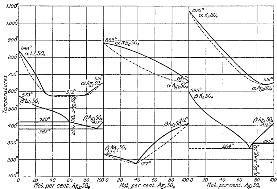
FIG. 20.—Binary System \text{Li}_2\text{SO}_4 — \text{Ag}_2\text{SO}_4 .
