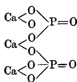
Ca_3(PO_4)_2
