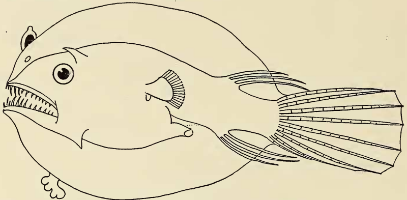
Fig. 27. Linophryne brevibarbata sp. nov. Post-larva.
