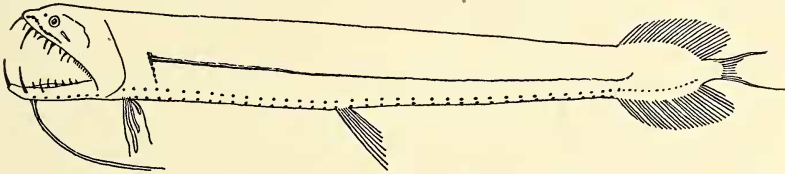
Fig. 9. Lamprotoxus angulifer sp. nov.
