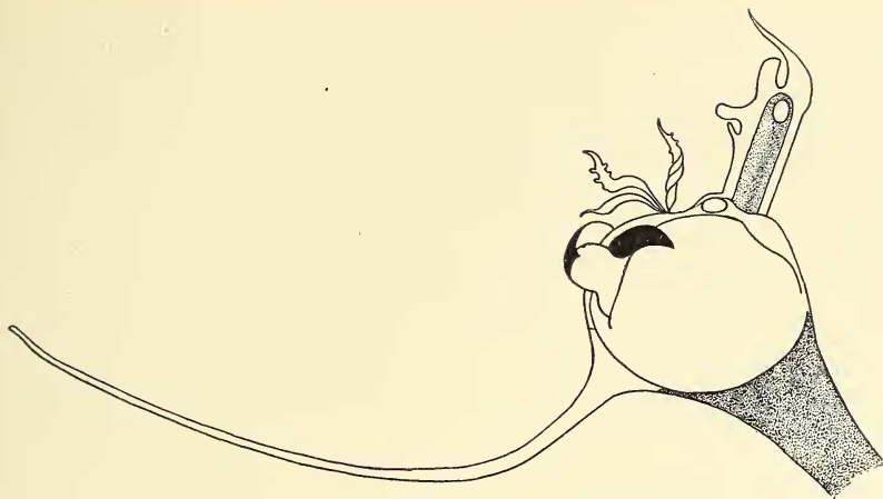
Fig. 23. Dolopichthys tentaculatus sp. nov.
