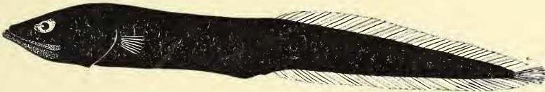
Fig. 20. Parabrotula dentiens sp. nov.
