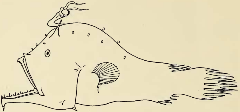
Fig. 28. Lophodolus lyra sp. nov.
