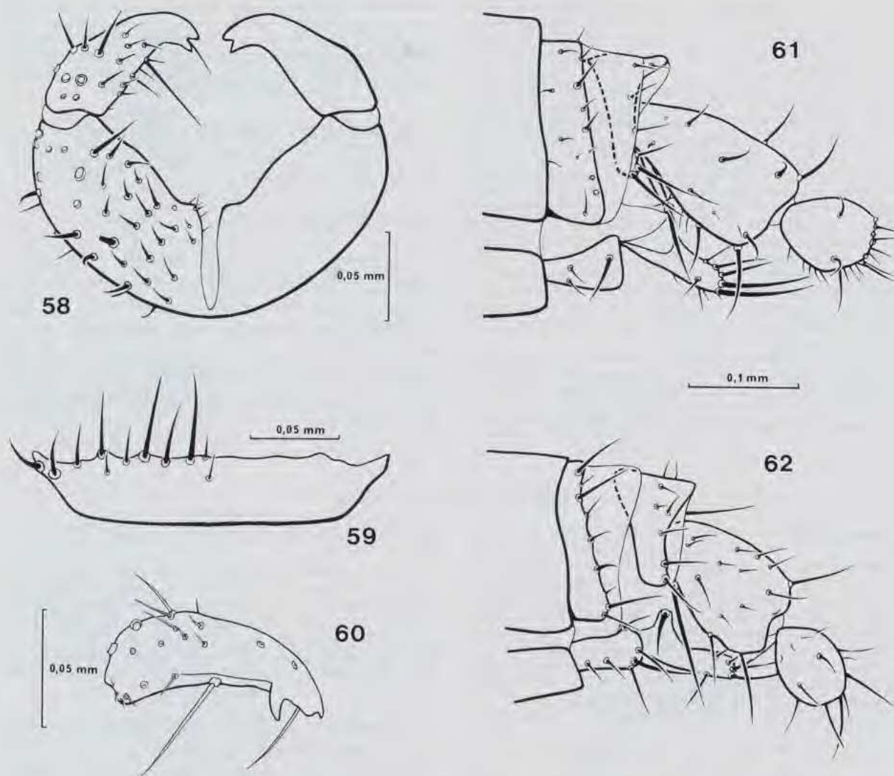
FIG. 58-62. — 58-60 : Tetragoneura usitata n. sp., holotype, hypopygè. 58 : face ventrale ; 59 : tergite IX ; 60 : gonostyle, vue paraventràle. 61-62 : Ovipositeur des Tetragoneura , holotypes, vue latérale. 61 : T. occulta n. sp. ; 62 : T. reducta n. sp.
