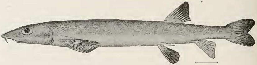
FIG. 5.—GONORHYNCHUS ABBREVIATUS
