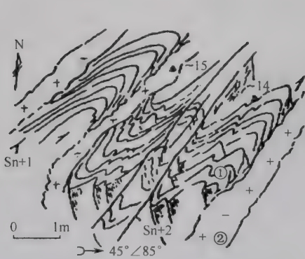
图9 瑞丽广喊回蚌韧性剪切带旁侧倾竖褶皱素描图
