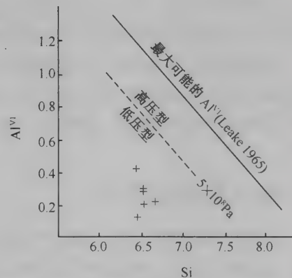
图7 表示角闪石压力型的 \text{Al}^{\text{VI}}-\text{Si} 变异图 (Raase 1974)
