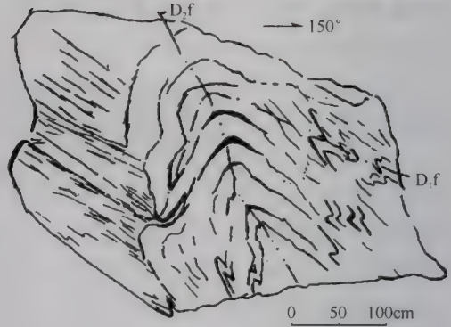
图10 瑞丽南京里 Pt_2gl^h 中共轴叠加褶皱
