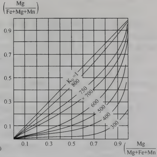
图5 变质岩中共存的 黑云母和石榴石之间 \text{Mg-Fe} 分配系数与 变质温度的关系 (Перчук 1970)
