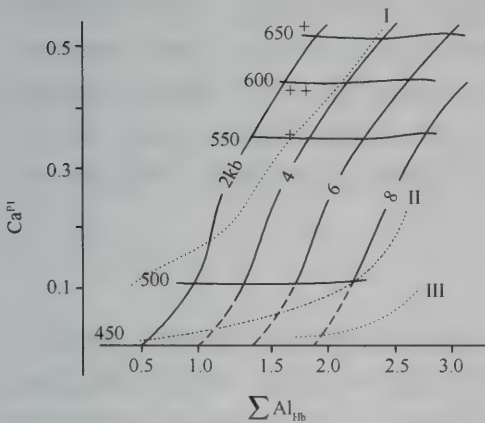
图6 斜长石-角闪石实验地质温 压计 (Plyusnina 1982)
