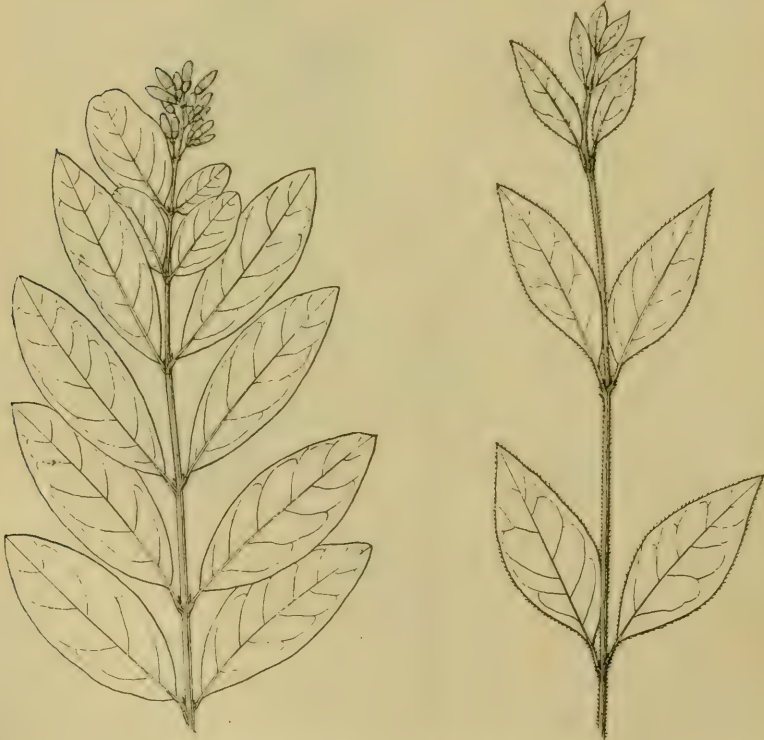
Fig. 81. Ligustrum Ibot , n. d. Nat. ( \frac{3}{4} ).
