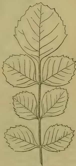
Fig. 25. Fraxinus rotundifolia , n. Willd. (2/4)
