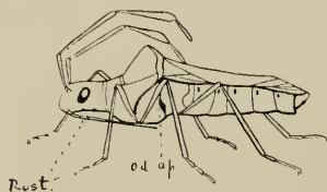
Fig. 435—HOMOCERUS. SCUT = SCUTELLUM. CLAV = CLAVUS. COR = CORIUM. ROST = ROSTRUM. OD. AP. = ODORIFEROUS APERTURES.
