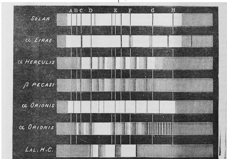
FIG. 5.—Various Stellar Spectra (Secchi).
