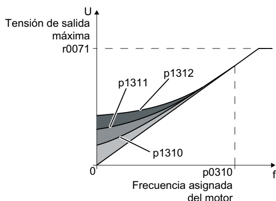
Figura 6-60 Elevación de la tensión resultante en el ejemplo de una característica lineal
