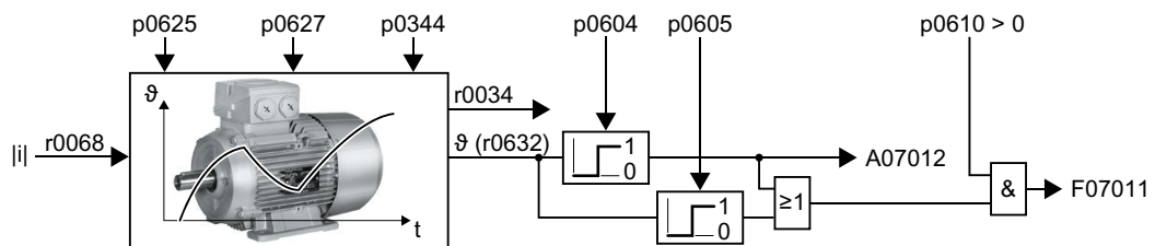
Figura 6-72 Modelo térmico de motor 2 para motores de inducción
