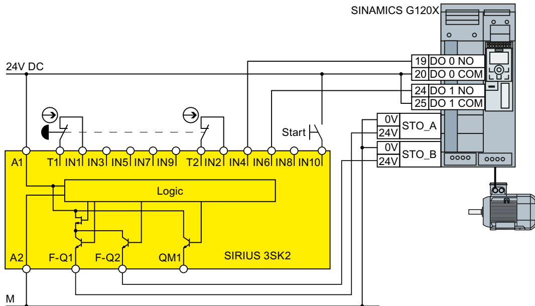
Figura 4-28 Conexión 3SK2 dentro de un armario eléctrico para FSA...FSG
