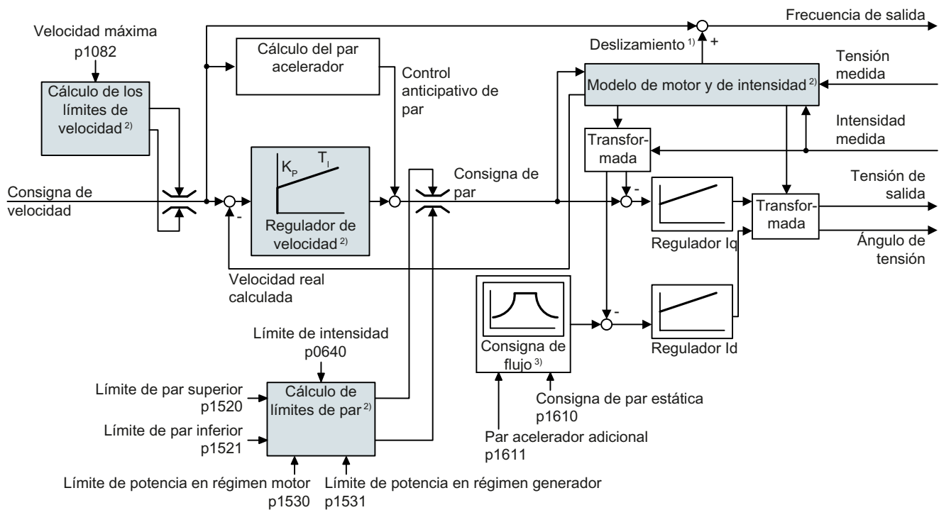
Figura 6-66 Esquema de funciones simplificado para regulación vectorial sin encóder con regulador de velocidad
