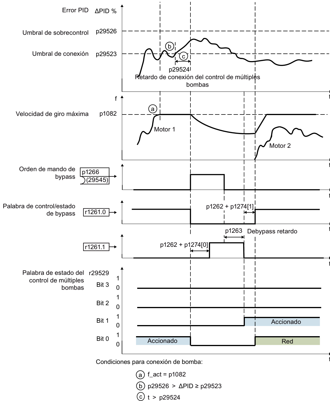
Figura 6-22 Conexión de bombas
