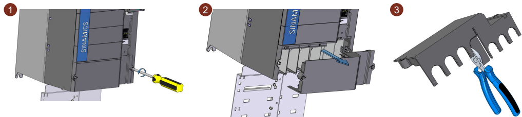
Figura 4-11 Retirada de la tapa de conexión y realización de orificios, FSF/FSG
