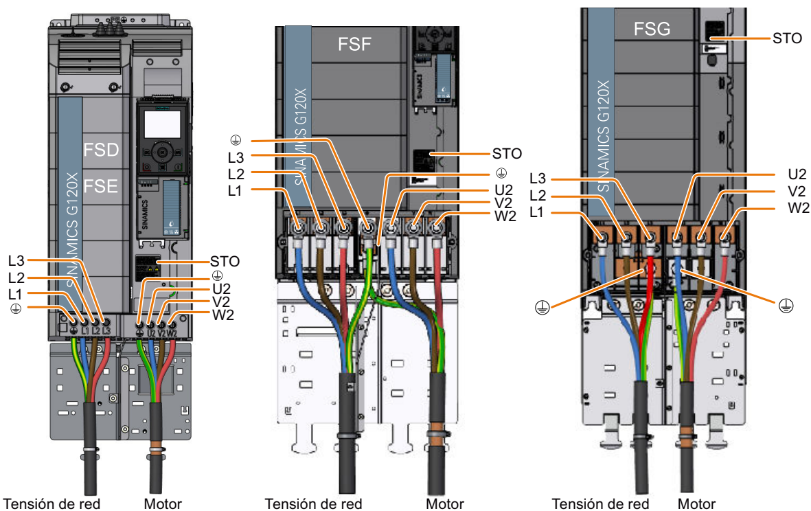
Figura 4-12 Conexiones de la alimentación de red y del motor
