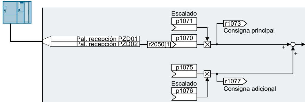
Figura 6-30 Bus de campo como fuente de consigna
