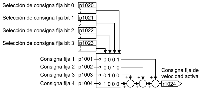
Figura 6-35 Selección directa de consignas fijas de velocidad
