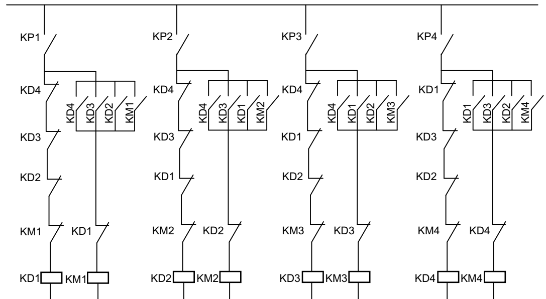
Figura 6-21 Circuito de control con relés externos
