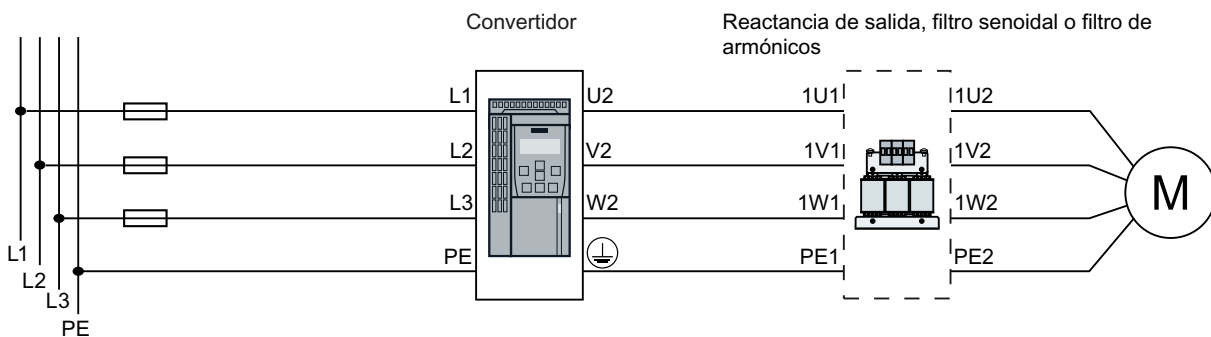
Figura 4-6 Conexión de convertidores FSD...FSG de 400 V y sus componentes opcionales
