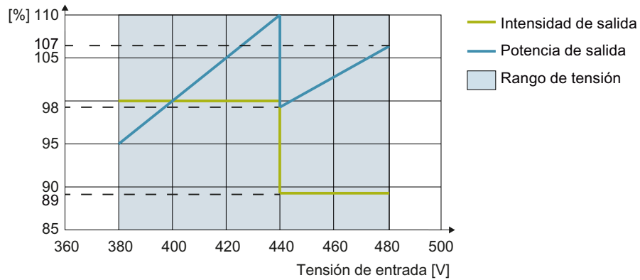
Figura 11-1 Reducción de intensidad y de tensión en función de la tensión de entrada para FSA ... FSG
