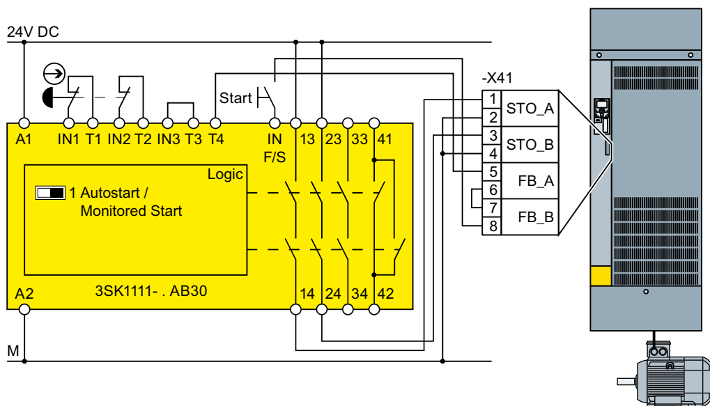
Figura 4-27 Conexión 3SK1 dentro de un armario eléctrico para FSH, FSJ
