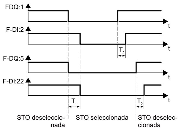
Figura 4-35 Vigilancia dinámica de la respuesta STO para FSA...FSG
