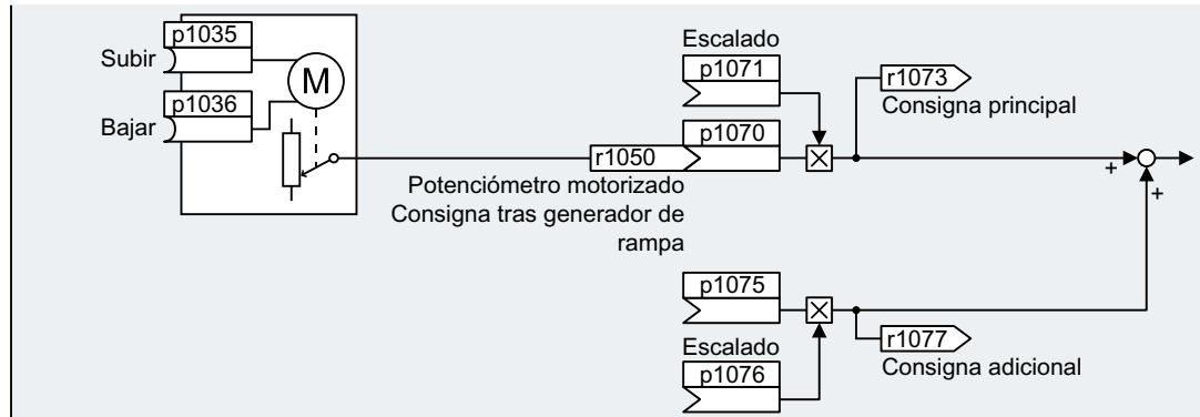
Figura 6-31 Potenciómetro motorizado como fuente de consigna
