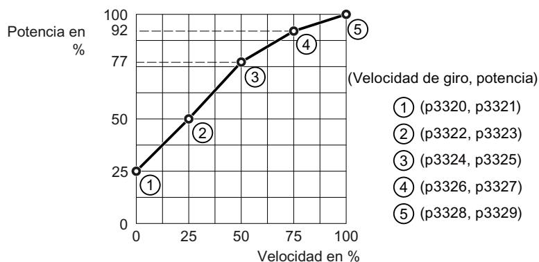
Figura 6-97 Ajuste de fábrica de la característica de flujo
