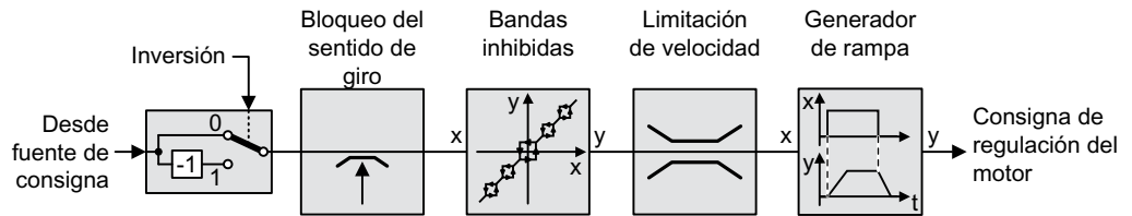
Figura 6-39 Acondicionamiento de consigna en el convertidor
