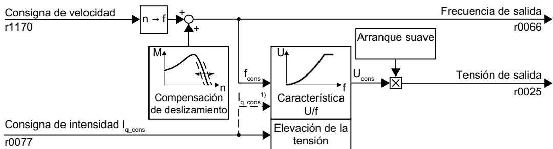
Figura 6-57 Esquema de funciones simplificado del control por U/f
