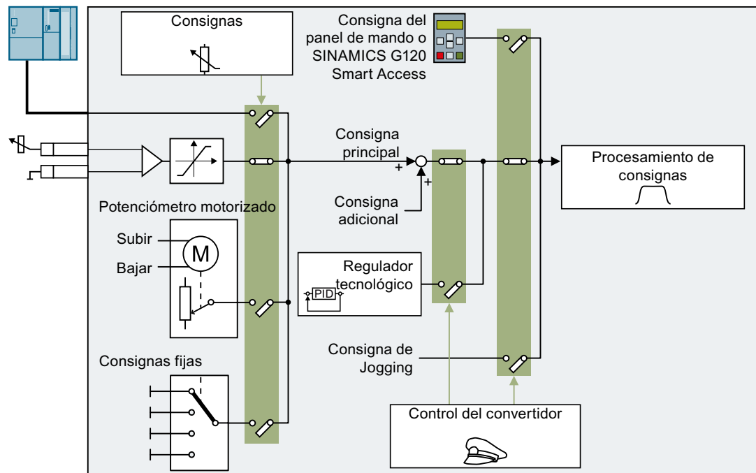
Figura 6-28 Fuentes de consignas para el convertidor
