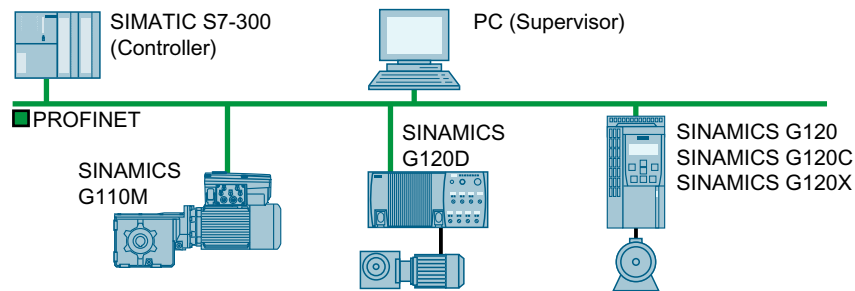
Figura 4-37 El convertidor en modo PROFINET IO
