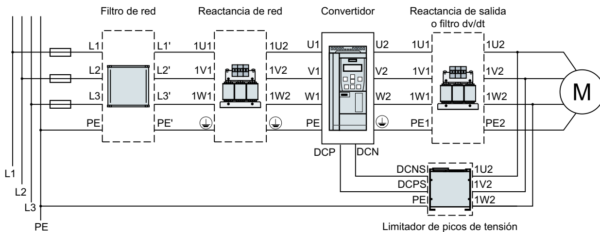
Figura 4-8 Conexión de convertidores FSH/FSJ y sus componentes opcionales
