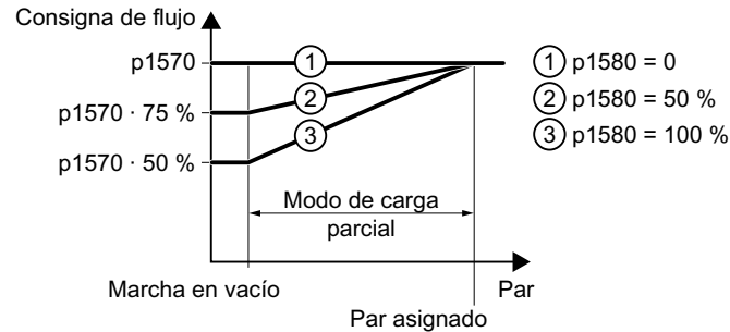
Figura 6-84 Reducción de la consigna de flujo en la zona de carga parcial del motor
