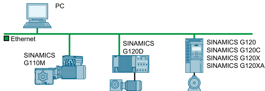
Figura 4-38 El convertidor como estación Ethernet
