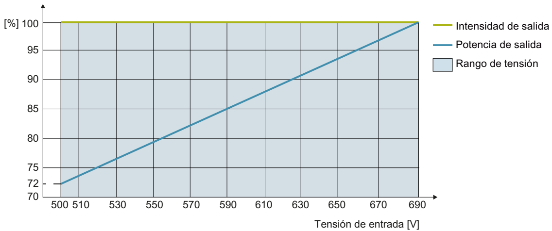
Figura 11-3 Reducción de intensidad y de tensión en función de la tensión de entrada para FSA ... FSG
