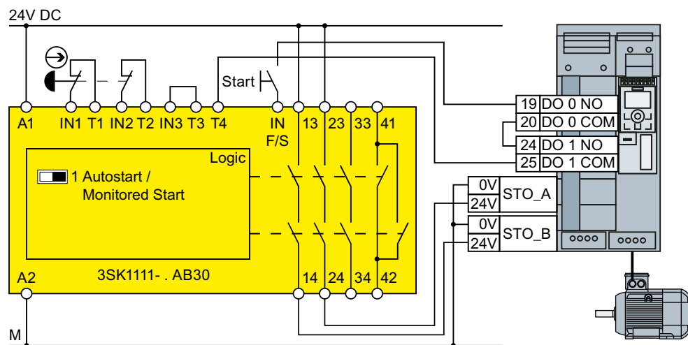
Figura 4-26 Conexión 3SK1 dentro de un armario eléctrico para FSA...FSG
