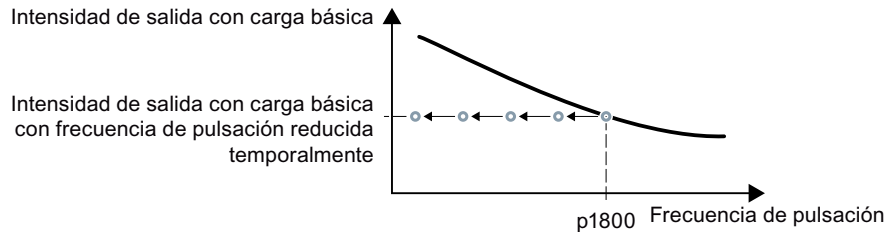
Figura 6-71 Característica de derating e intensidad de salida para carga básica en caso de sobrecarga
