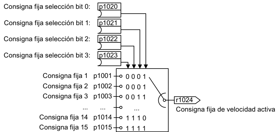
Figura 6-36 Selección binaria de consignas fijas de velocidad
