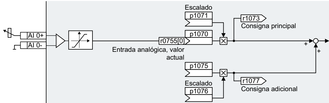
Figura 6-29 Ejemplo: entrada analógica 0 como fuente de consigna
