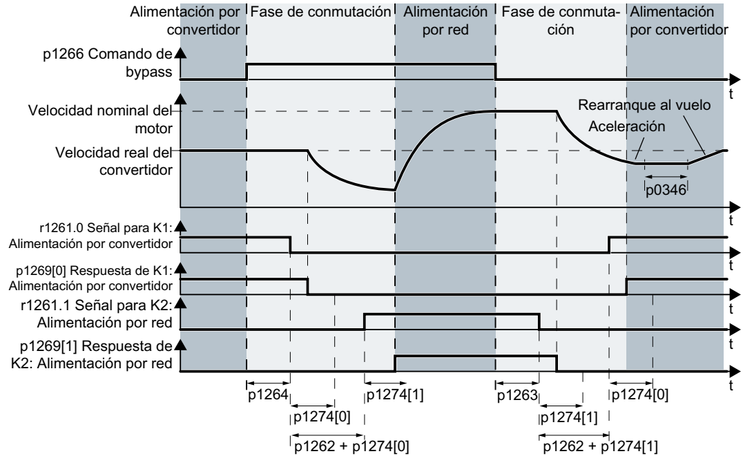
Figura 6-87 Conmutación activada mediante una señal de mando (p1267.0 = 1)
