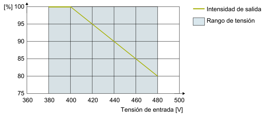
Figura 11-2 Reducción de intensidad en función de la tensión de entrada para FSH/FSJ
