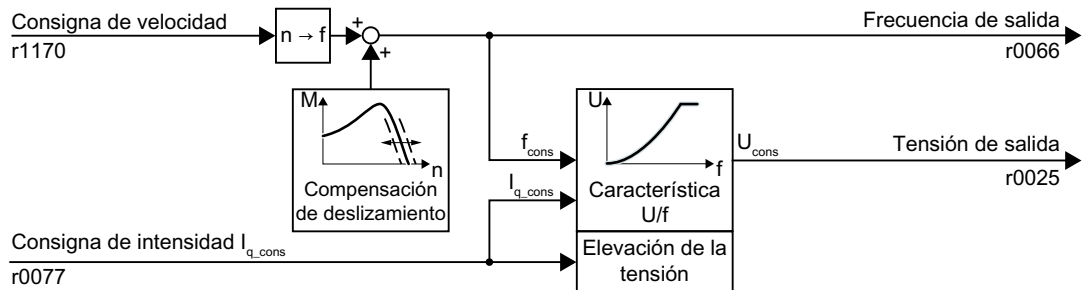
Figura 6-63 Ajuste predeterminado del control por U/f tras elegir Standard Drive Control
