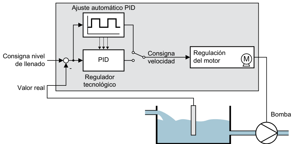
Figura 6-48 Ajuste automático según el ejemplo de una regulación de nivel
