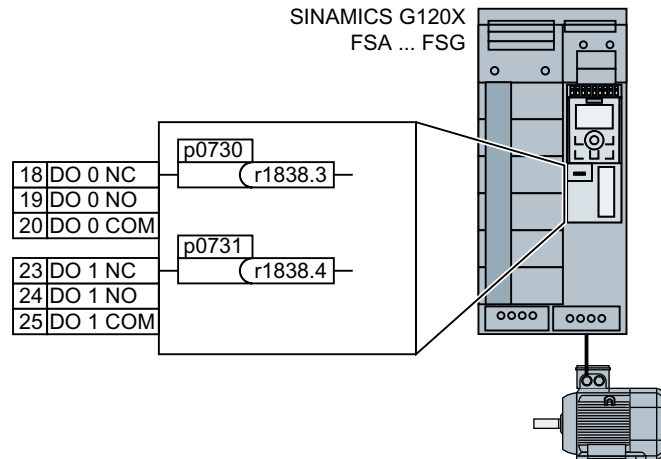
Figura 6-19 Respuesta "STO activo" a través de las salidas digitales
