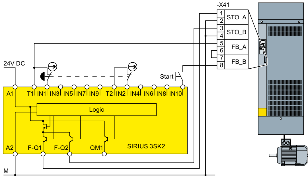
Figura 4-30 Conexión 3SK2 dentro de un armario eléctrico para FSH y FSJ
