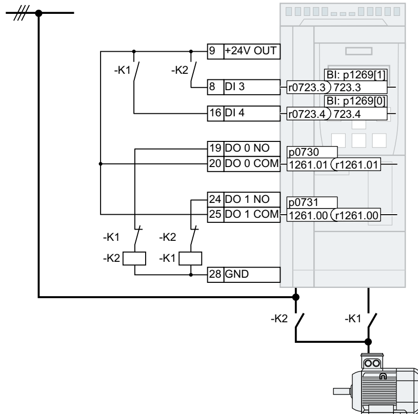
Figura 6-86 Control de bypass a través del convertidor
