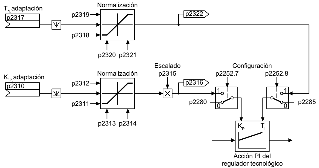
Figura 6-50 Adaptación del regulador
