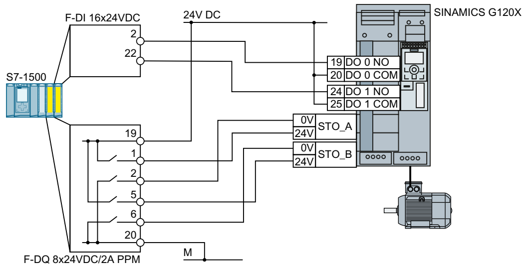
Figura 4-34 Conexión de SIMATIC S7-1500 dentro de un armario eléctrico para FSA...FSG
