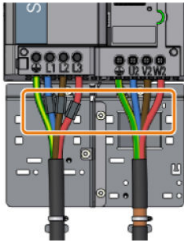
Figura 4-4 Anillos de ferrita en los cables de conexión
