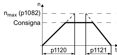
Figura 5-12 Tiempos de aceleración y deceleración del motor
