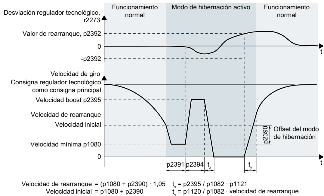
Figura 6-90 Modo de hibernación vía consigna tecnológica como consigna principal con boost
