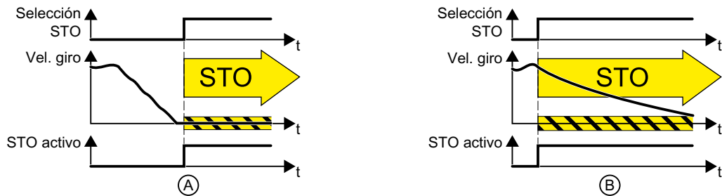
Figura 6-18 Funcionalidad de STO cuando el motor está en parada (A) y en giro (B)
