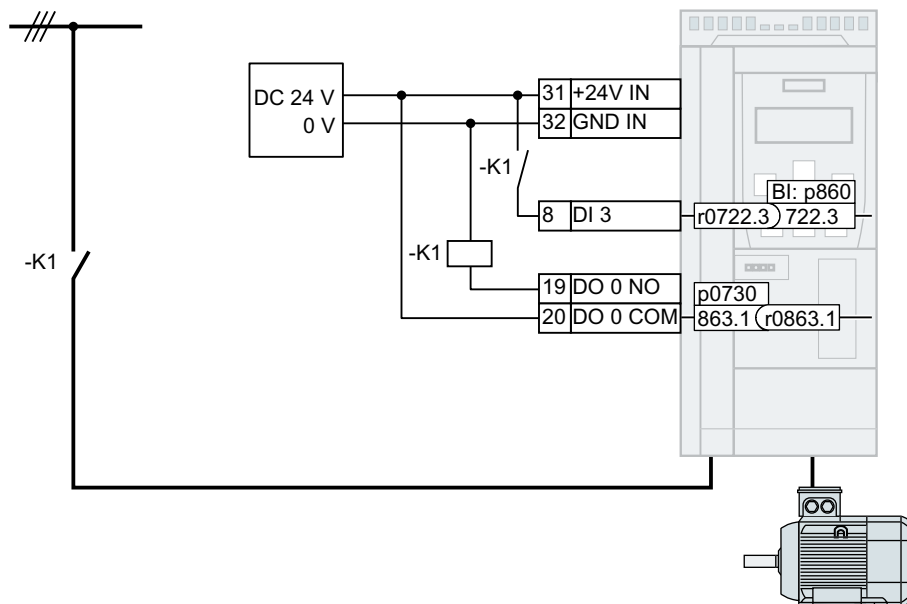
Figura 6-93 Control del contactor de red a través de DO 0 con respuesta a través de DI 3
