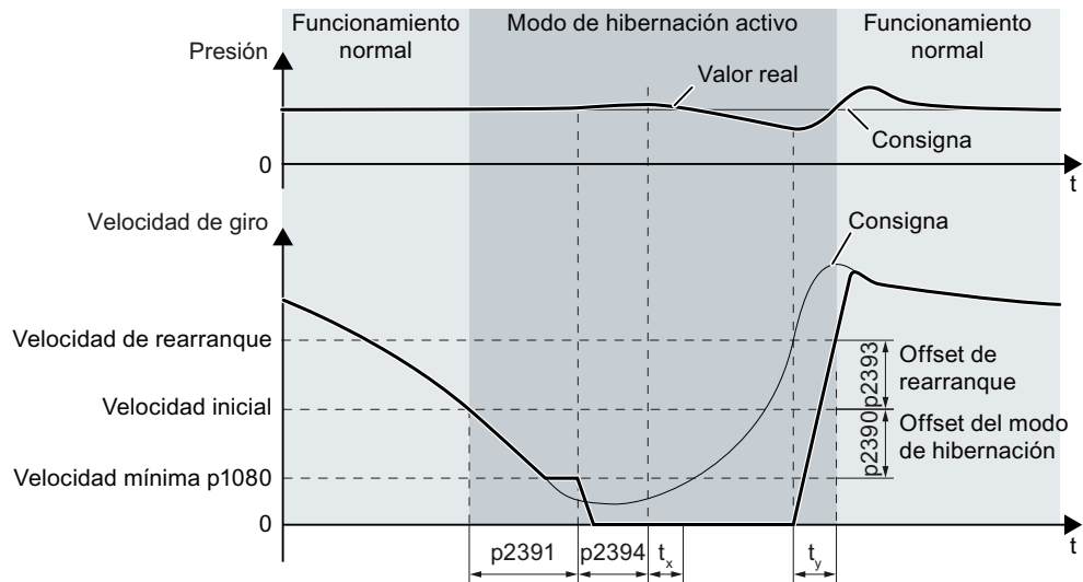
Figura 6-91 Modo de hibernación vía consigna externa con boost
