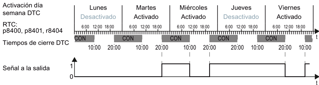
Figura 6-56 Ejemplo de comportamiento del programador horario
