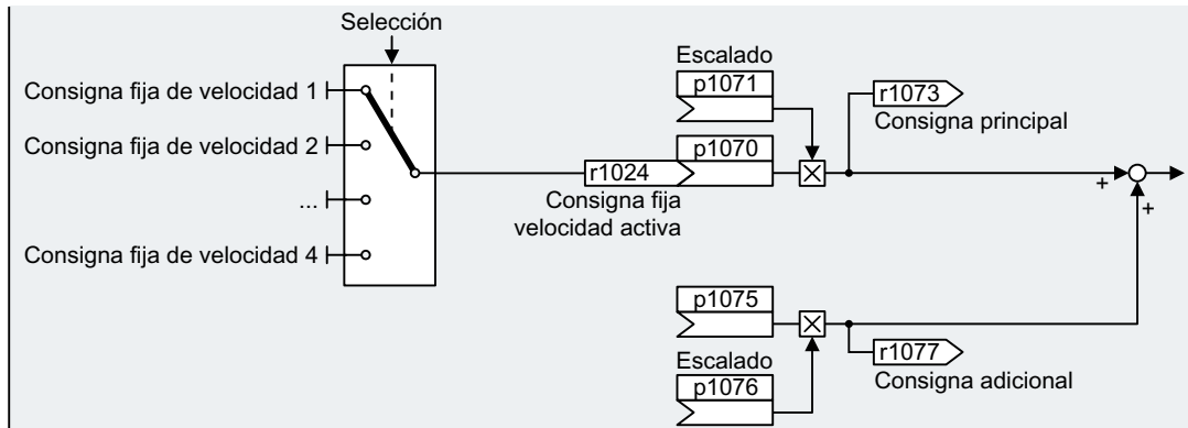
Figura 6-34 Consigna fija de velocidad como fuente de consigna
