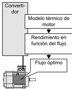
Figura 6-82 Cálculo del flujo óptimo a partir del modelo térmico del motor
