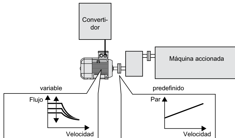
Figura 6-81 Optimización de rendimiento mediante cambio del flujo del motor
