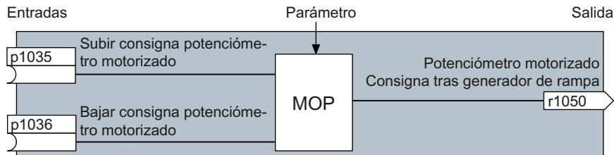
Figura A-3 Ejemplo de bloque: Potenciómetro motorizado (PMot)
