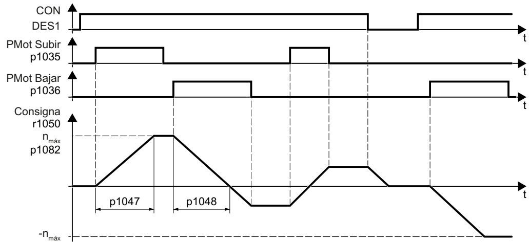
Figura 6-32 Diagrama funcional del potenciómetro motorizado
