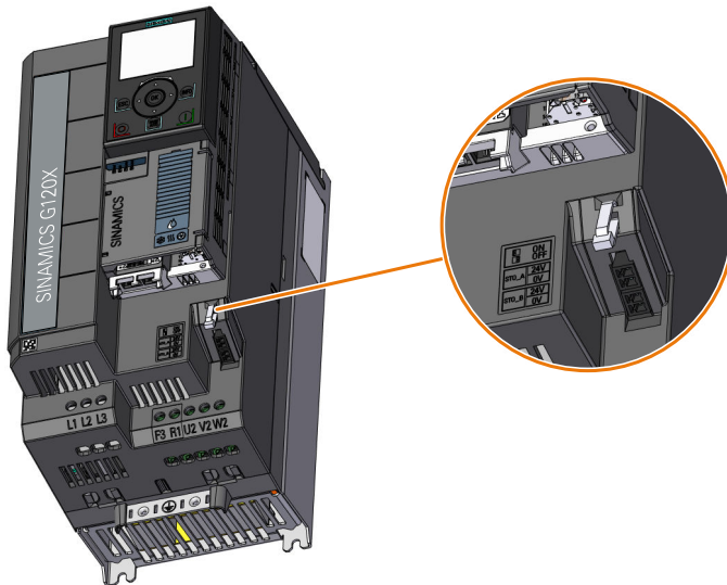
Figura 4-25 Protección contra la inhibición accidental de la función "STO", FSA ... FSC
