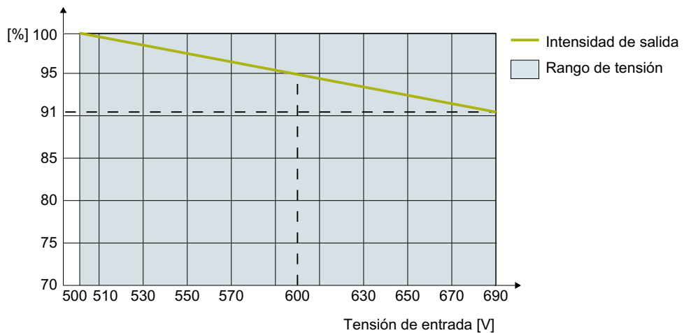
Figura 11-4 Reducción de intensidad en función de la tensión de entrada para FSH/FSJ
