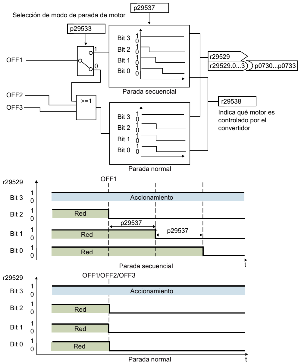
Figura 6-25 Modo de parada
