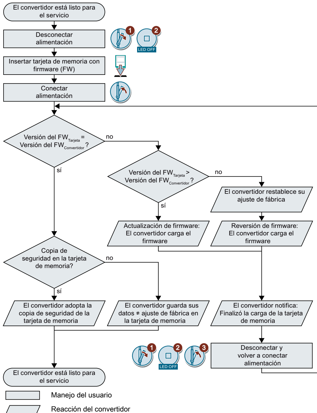
Figura 10-2 Resumen de la actualización y la reversión del firmware
