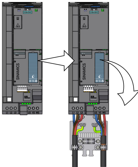
Figura 10-1 Sustitución de un convertidor defectuoso
