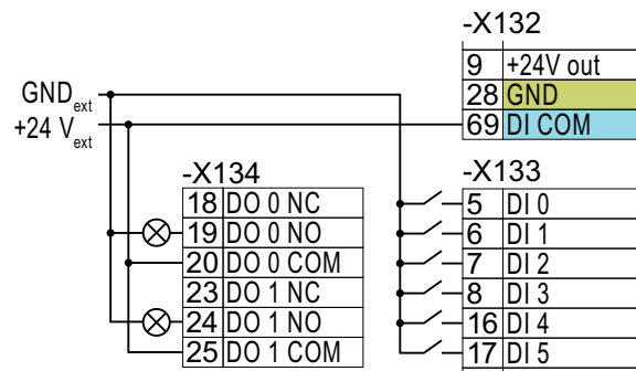
Figura 4-17 Conexión de contactos que conmutan a potencial m con una alimentación externa
