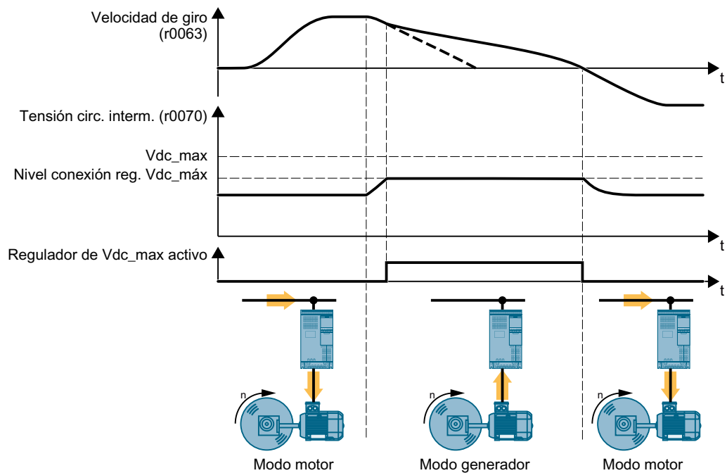
Figura 6-74 Representación simplificada de la regulación de V_{dc\_máx}
