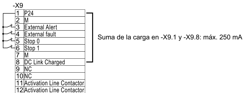
Figura 4-21 Regleta de bornes X9 con alimentación interna de 24 V
