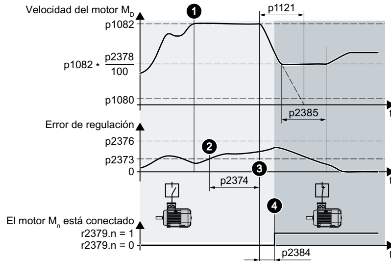
Figura 6-54 Activar motores no regulados M_1 \dots M_2
