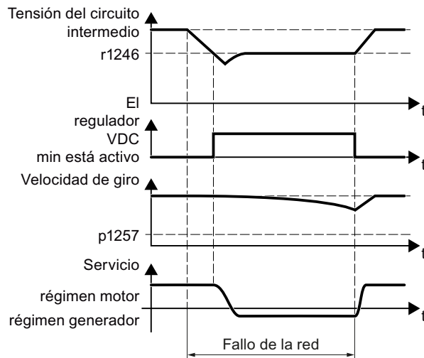
Figura 6-79 Funcionamiento básico del respaldo cinético
