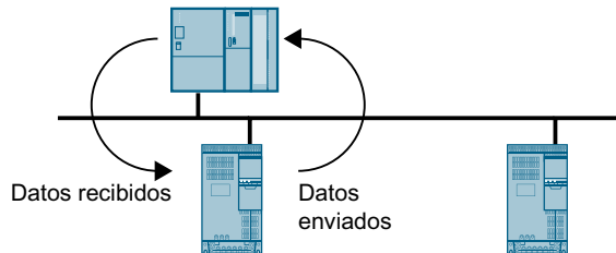
Figura 6-10 Intercambio de datos cíclico
