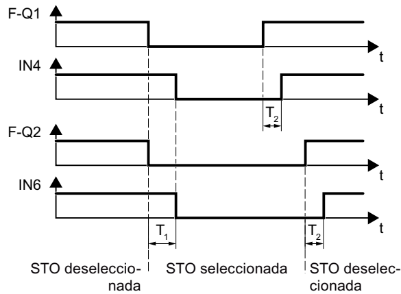
Figura 4-29 Vigilancia dinámica de la respuesta STO para FSA...FSG
