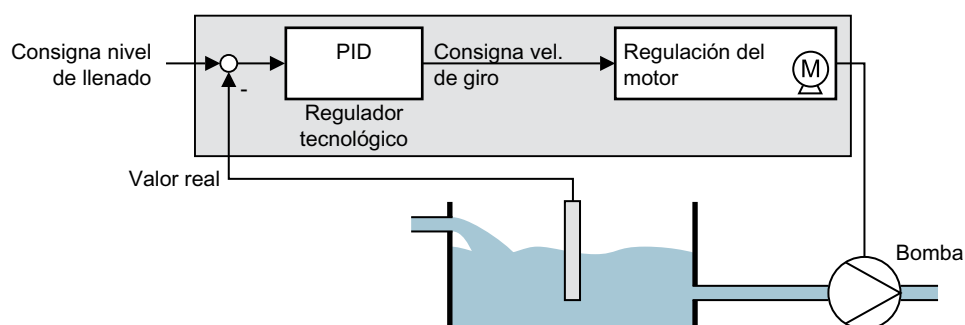
Figura 6-42 Ejemplo de regulador tecnológico como regulador de nivel
