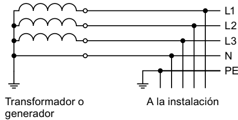
Figura 4-2 Sistema TT
