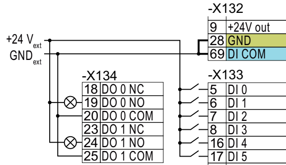
Figura 4-16 Conexión de contactos que conmutan a potencial p con una alimentación externa
