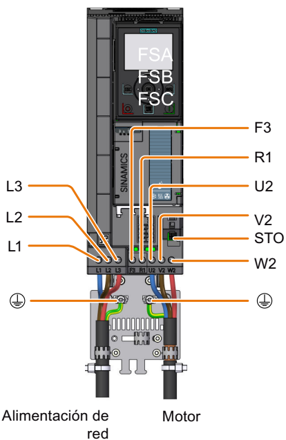
Figura 4-9 Conexiones para la alimentación de red, motor y bornes del circuito intermedio de DC
