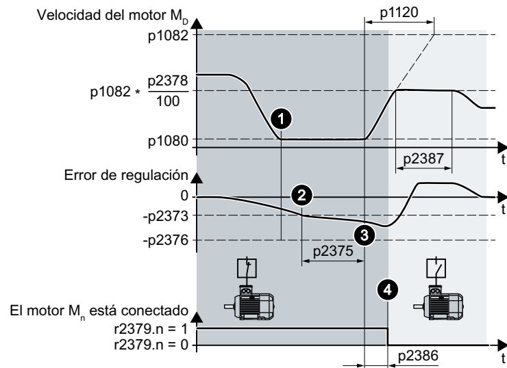
Figura 6-55 Desactivar motores no regulados M 1 ... M 2
