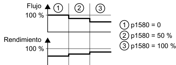
Figura 6-85 Resultado cualitativo de la optimización de rendimiento, método 1
