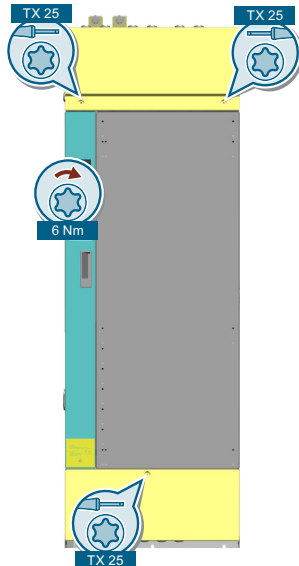
Figura 4-13 Desmontaje de la cubierta frontal
