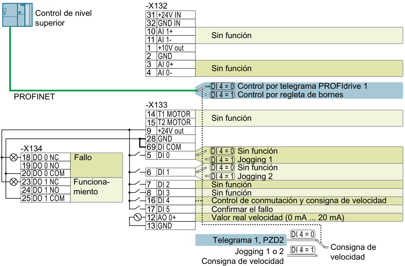
Figura 4-18 Ajustes de fábrica de la interfaz
