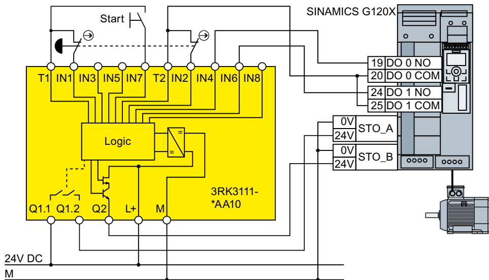
Figura 4-31 Conexión 3RK3 dentro de un armario eléctrico para FSA...FSG
