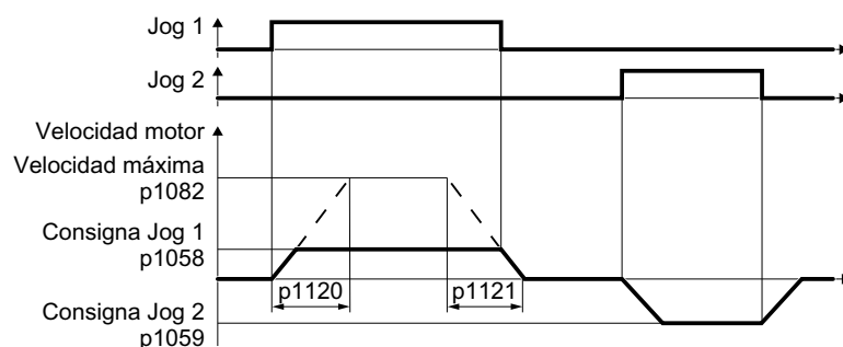
Figura 6-17 Comportamiento del motor con "JOG"
