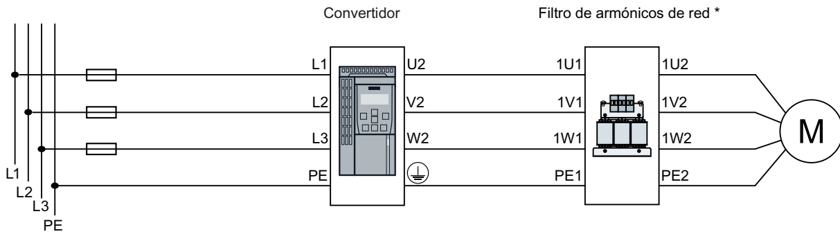
Figura 4-5 Conexión de convertidores FSA...FSC y sus componentes opcionales
