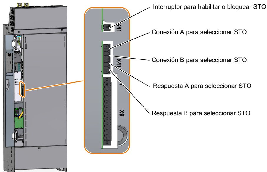
Figura 4-24 Bornes e interruptores para la función "STO", tamaños FSH y FSJ
