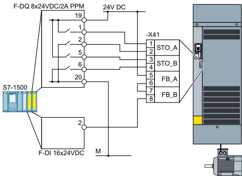
Figura 4-36 Conexión de SIMATIC S7-1500 dentro de un armario eléctrico para FSH y FSJ
