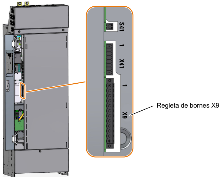
Figura 4-19 Regleta de bornes X9
