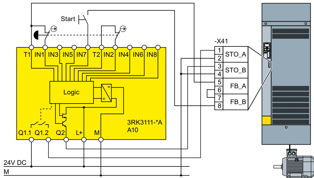
Figura 4-33 Conexión 3RK3 dentro de un armario eléctrico para FSH y FSJ
