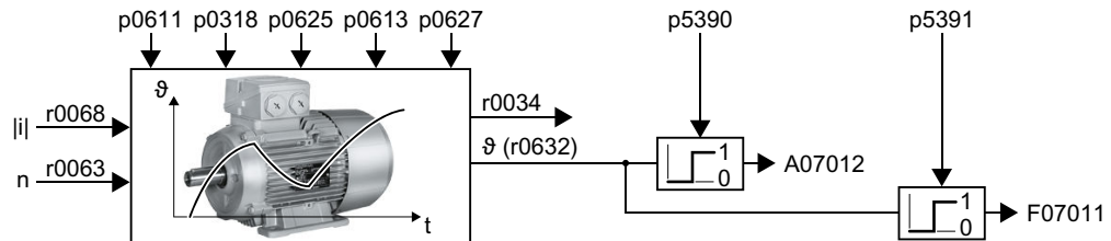
Figura 6-73 Modelo térmico de motor 1 para motores de reluctancia
