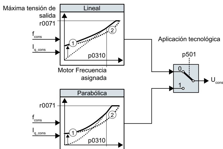
Figura 6-64 Características tras elegir Standard Drive Control
