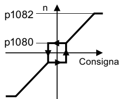
Figura 5-11 Velocidades mínima y máxima del motor
