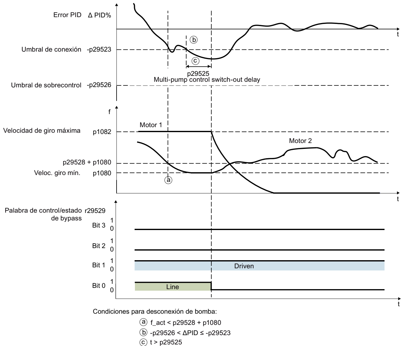
Figura 6-24 Desconexión de bombas según las horas absolutas de funcionamiento (p29522 = 1)
