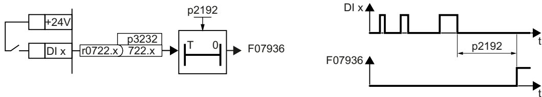
Figura 6-75 Esquema de funciones y comportamiento en el tiempo de la vigilancia de giro
