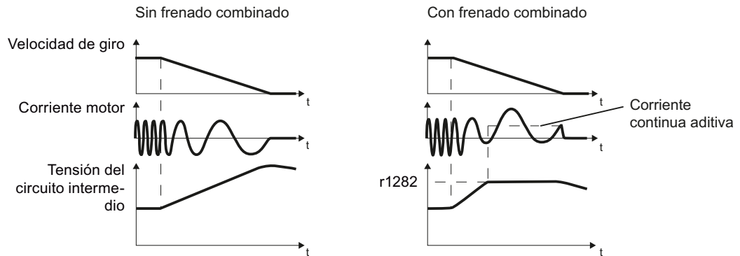
Figura 6-70 Frenado del motor con y sin frenado combinado activo
