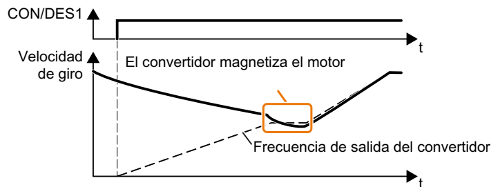
Figura 6-76 Funcionamiento básico de la función "Rearranque al vuelo"
