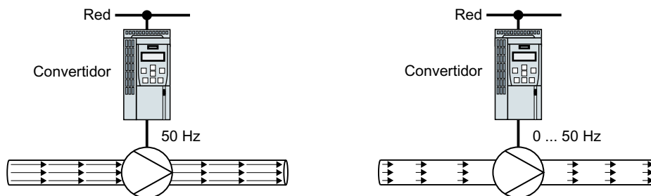
Figura 6-96 Regulación de flujo con bomba y convertidor
