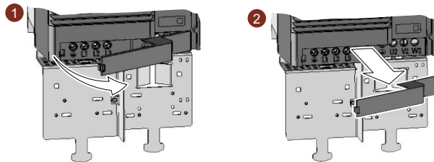
Figura 4-10 Retirada de la tapa de conexión, FSD/FSE
