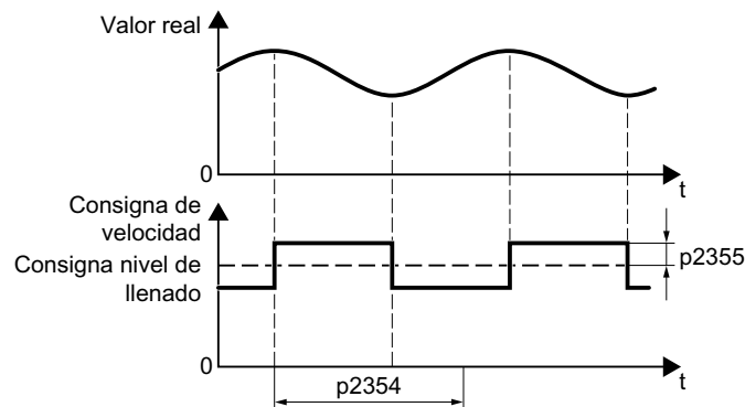
Figura 6-49 Ejemplo de consigna de velocidad y valor real de proceso en el ajuste automático
