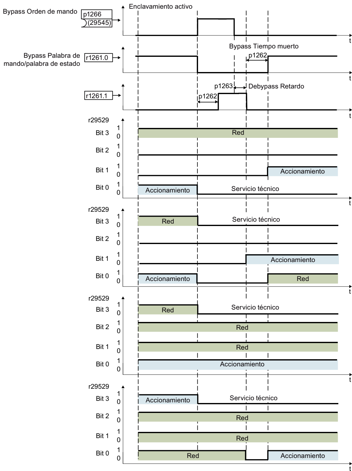
Figura 6-27 Modo de servicio
