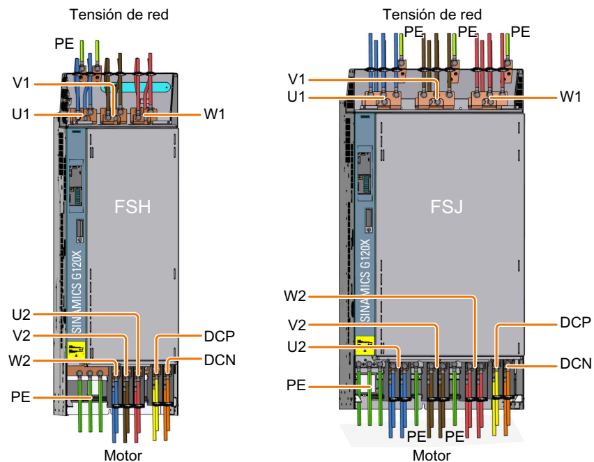
Figura 4-14 Conexiones para red, motor y circuito intermedio
