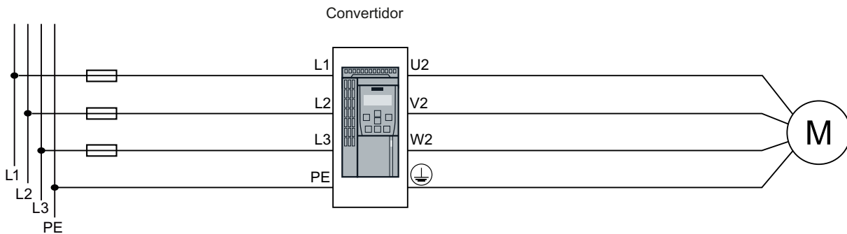
Figura 4-7 Conexión de convertidores FSD...FSG de 690 V y sus componentes opcionales
