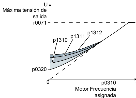
Figura 6-65 Elevación de la tensión resultante en el ejemplo de una característica lineal
