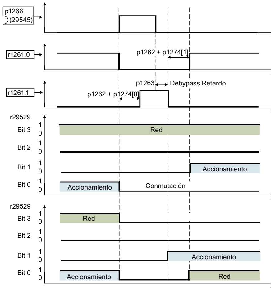
Figura 6-26 Conmutación de bombas
