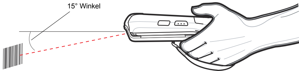
Abbildung 4-1 Linearscanner
