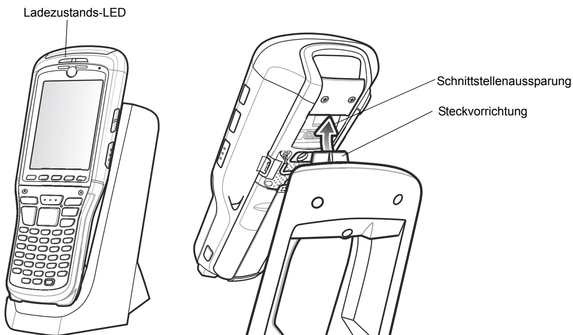
Abbildung 8-2 Akkuladevorgang beim MC9500-K
