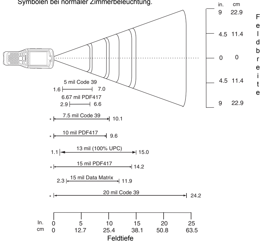
Abbildung 4-8 MC9500-K Imager-Decodierbereiche
