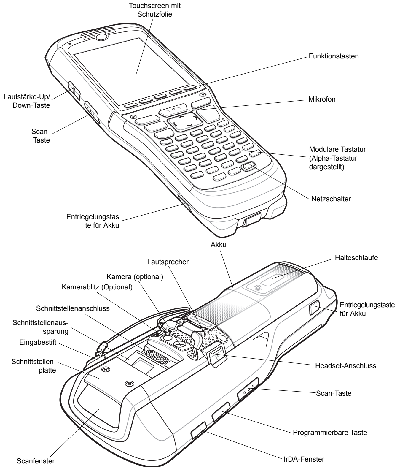
Abbildung 1-1 MC9500-K
