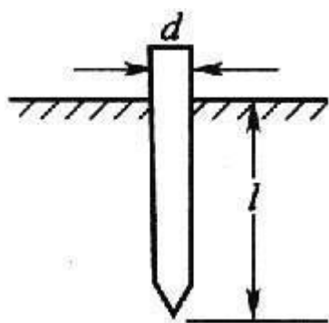
图 A.0.1—1 垂直接地极的示意
