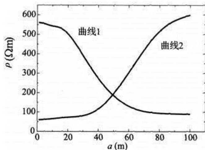
图 2 双层土壤的典型视在电阻率曲线
