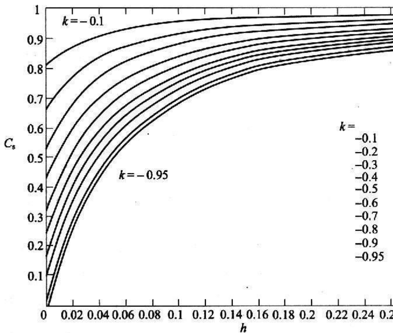
图 C.0.1 C_s 与 h 和 K 的关系曲线
