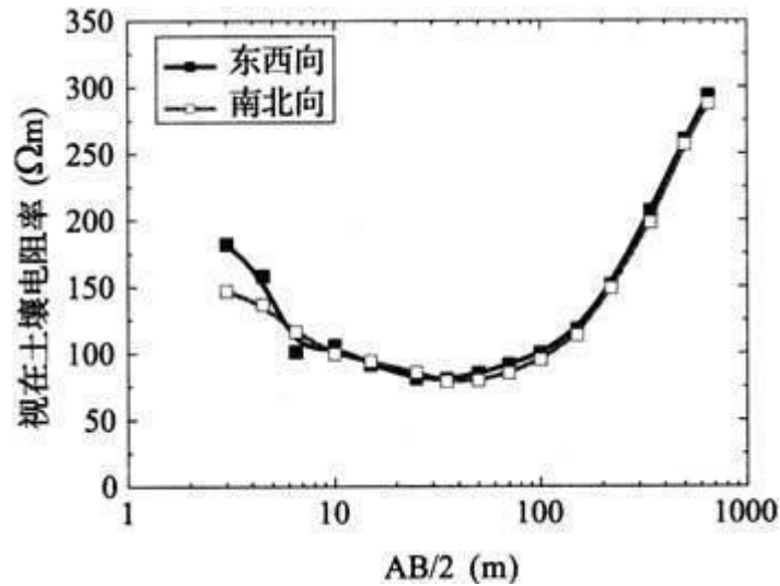
图 5 视在土壤电阻率测试结果
