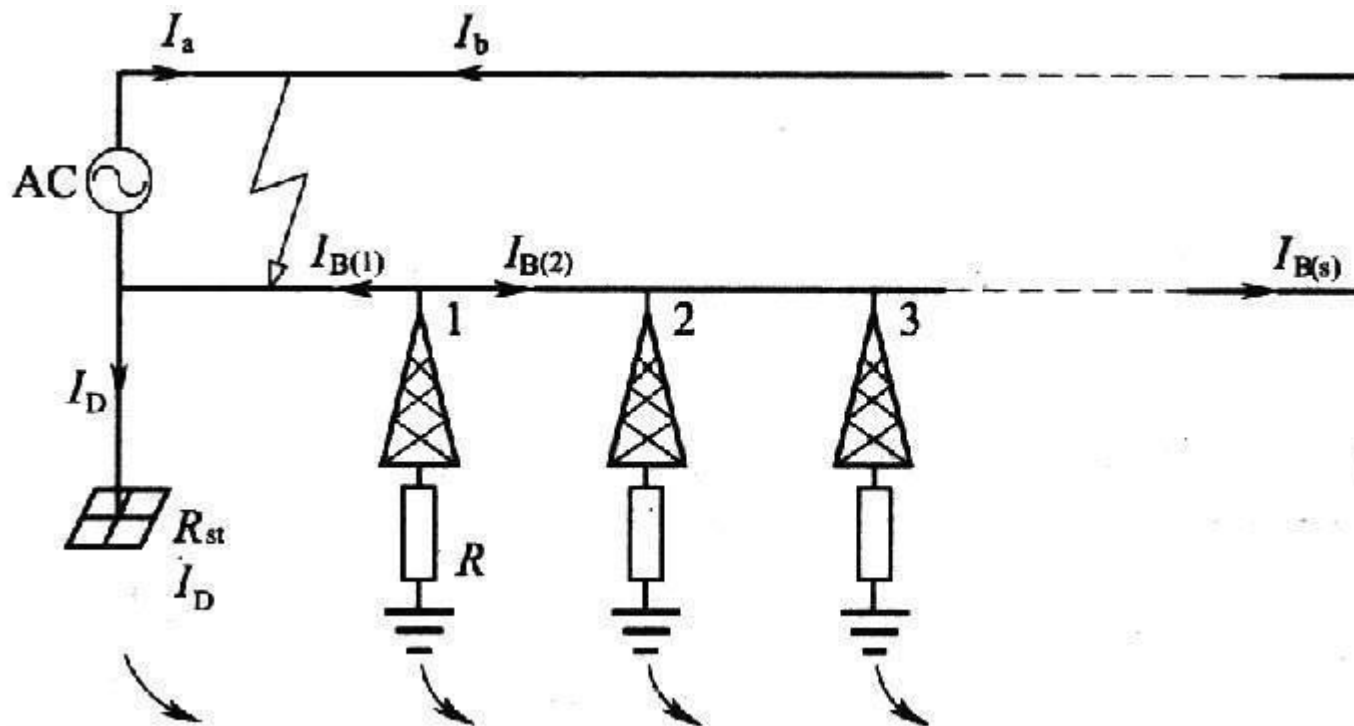
图 B.0.2—1 站内接地故障示意
