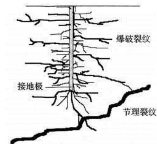
图 9 单根垂直接地极采用深孔爆破接地技术后形成的填充了降阻剂的区域
