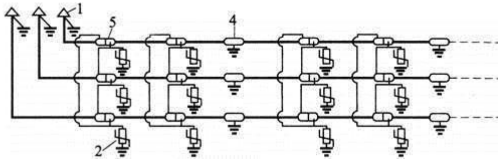
(c)交叉互联接地方式
