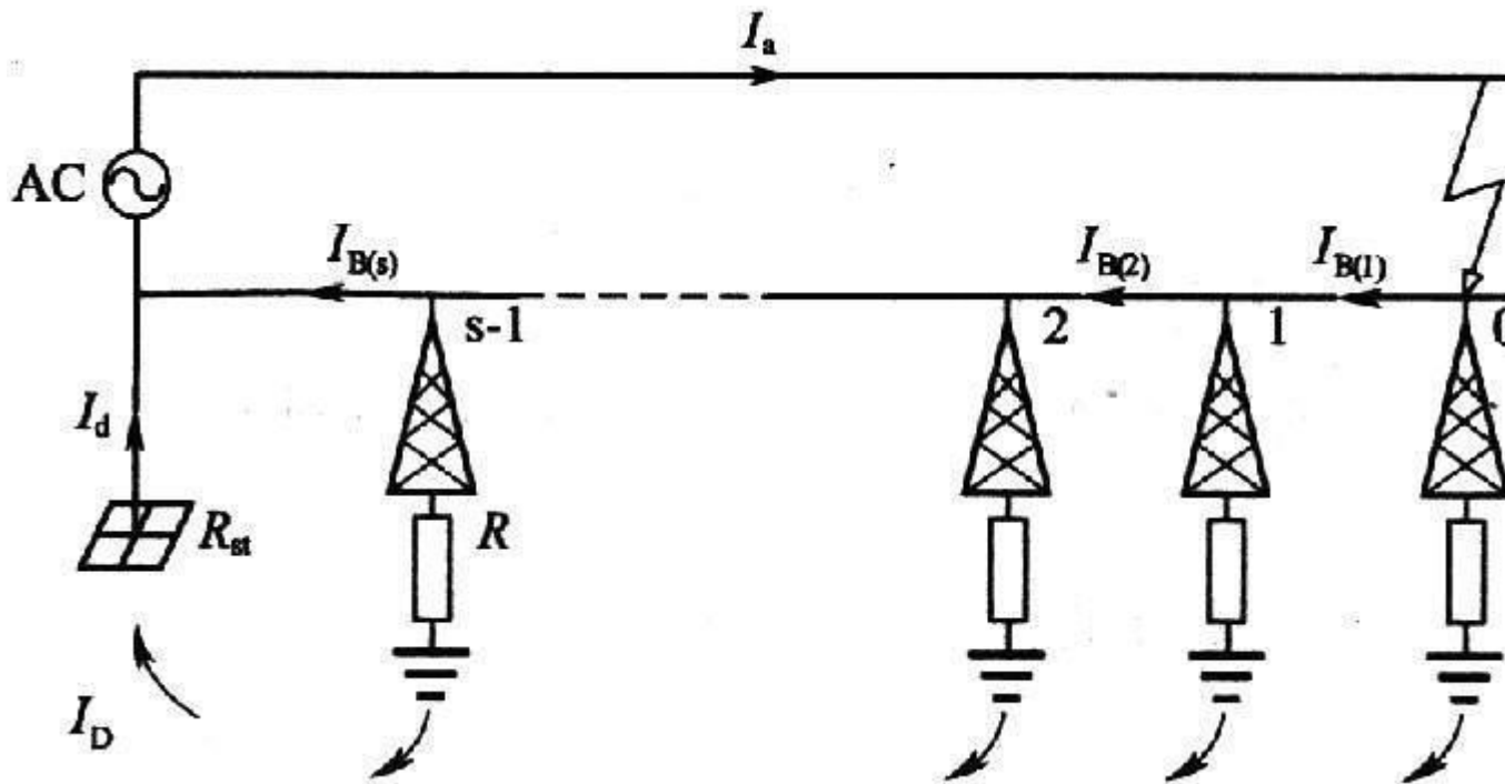
图 B.0.2—2 站外接地故障示意
