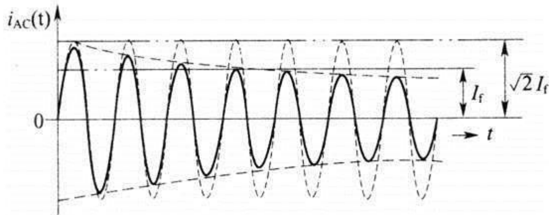
(a)对称分量
