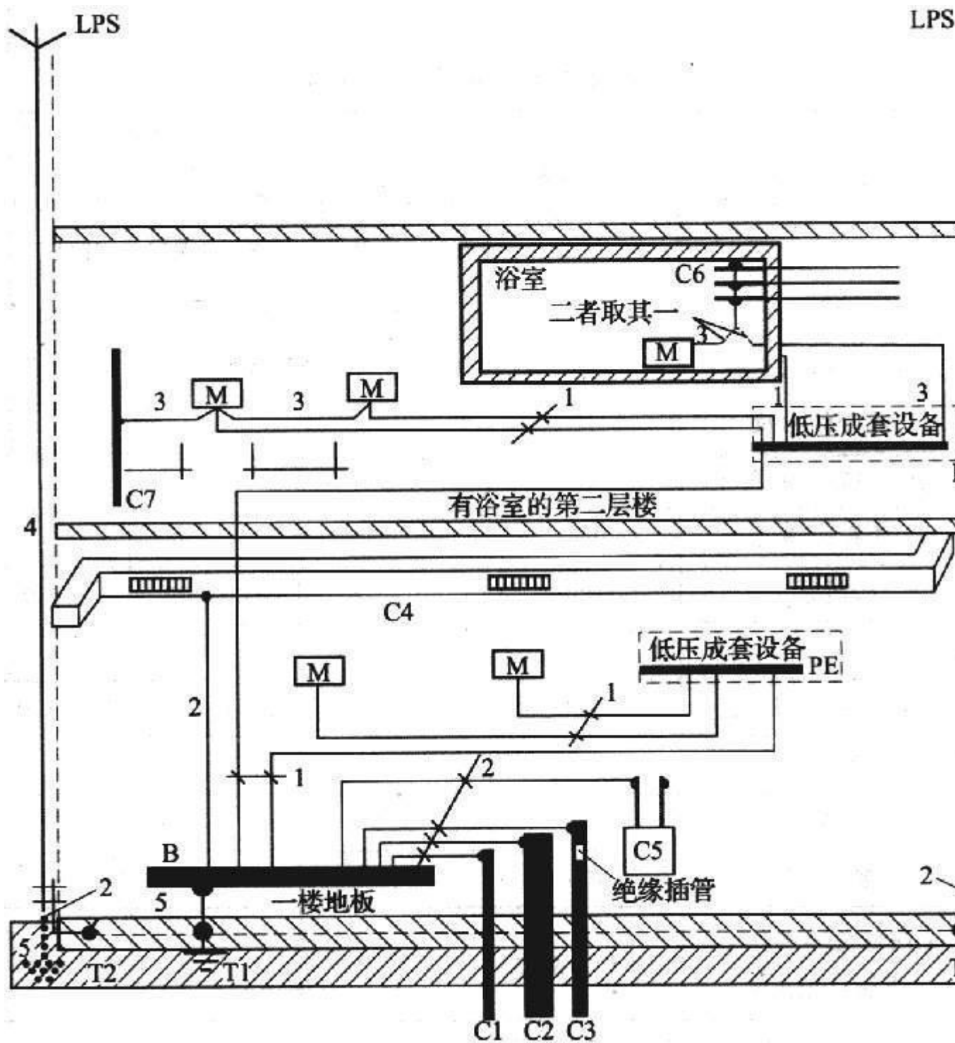
图 H 接地配置、保护导体和保护联结导体
