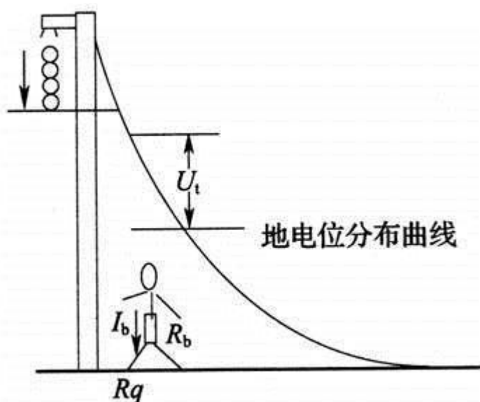
图 7 人体遭受接触电位差
