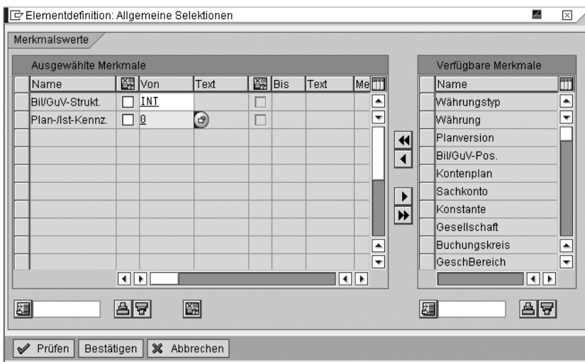
Abbildung 8.5 »Allgemeine Selektionen«
