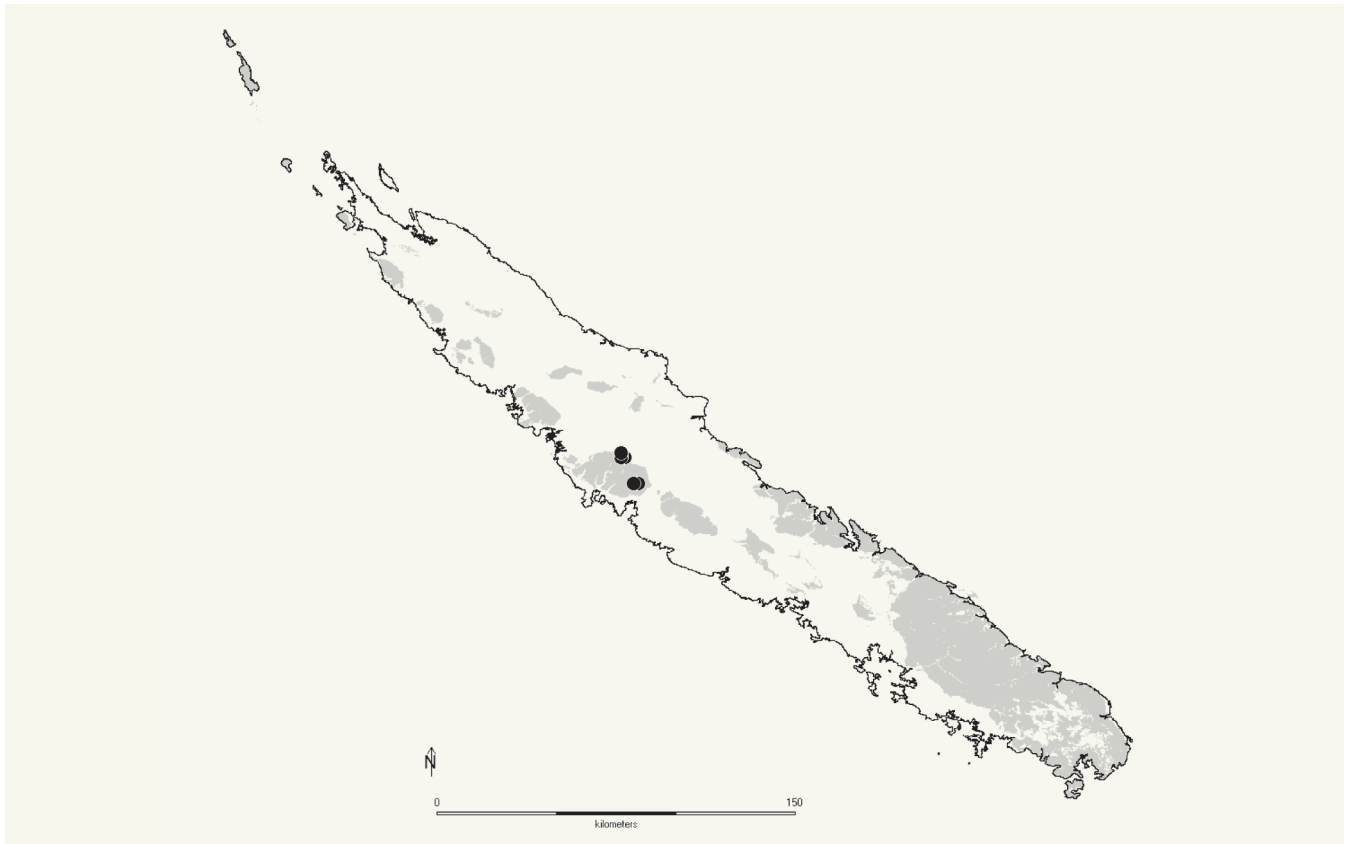
Fig. 3. – Distribution de Phelline barrieri Barriera & Schlüssel sur la Grande Terre, en gris les zones à roches ultramafiques.
