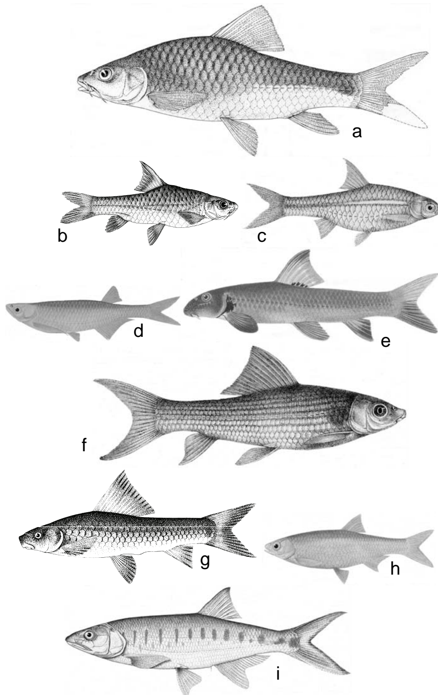
Figure 8. CYPRINIDAE: a. ' Barbus ' altianalis ; b. ' Barbus ' cercops (after Boulenger, 1909); c. ' Barbus ' magdalenae (after Boulenger, 1911); d. Chelaethiops bibie ; e. Garra dembeensis (after Boulenger, 1911), f. Labeo horie , g. Labeo victorianus ; h. Leptocypris niloticus (after Boulenger, 1911); i. Raiamas senegalensis .
