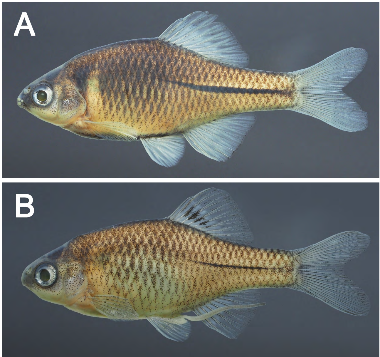
Fig. 1. Rhodeus cyanorostris sp. nov. A) SOU 1801001, holotype, ♂, 32.1 mm SL; B) SOU 1801004, paratype, ♀, 28.2 mm SL.
