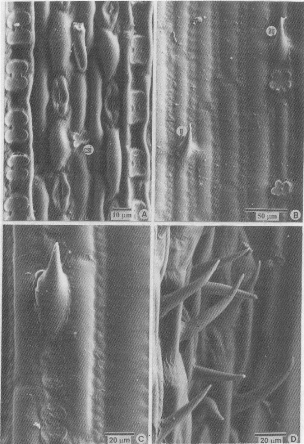
Fig. 4. Fotos de la epidermis foliar con MEB. A, epidermis abaxial de Schizachyrium salzmanni (Carnevali 3795) zonas costales laterales delimitan la zona intercostal central con células papilosas interestomáticas. B, C y D, epidermis adaxial en S. sanguineum (Quarín 3348) B, detalle de ganchos intercostales y aguijones costales correspondientes con haces de tercer orden ; C, aguijón costal; D, macropelos en la zona de la quilla o vena media. Abreviaturas: csi: cuerpo silíceo (4-lobulado), g: ganchos intercostales, ag: aguijones costales.
