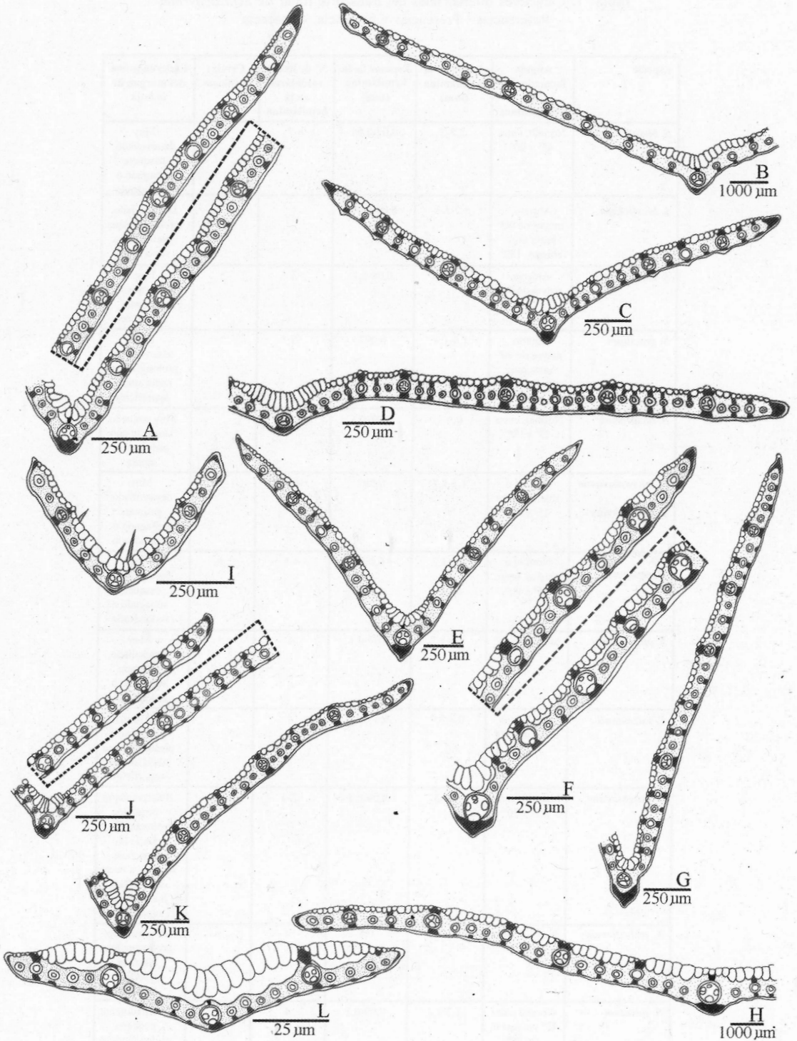
Fig. 1. Esquemas de transcortes foliares o de hemiláminas. A, Schizachyrium bimucronatum (Peichoto 12); B, S. brevifolium (Sulekic 816); C, S. condensatum (Vanni et al. 4591); D, S. gracilipes (Norrman 278); E, S. lactiflorum (Arbo et al. 8829); F, S. microstachyum ssp. microstachyum (Peichoto 11); G, S. plumigerum (Pedelabörde (SI 12168)); H, S. salzmannii (Peichoto 29); I, S. sanguineum (Peichoto & Schinini 7); J, S. scabriflorum (Vanni et al. 4603); K, S. spicatum (Cristóbal et al. 1669); L, S. tenerum (Peichoto & Schinini 9).
