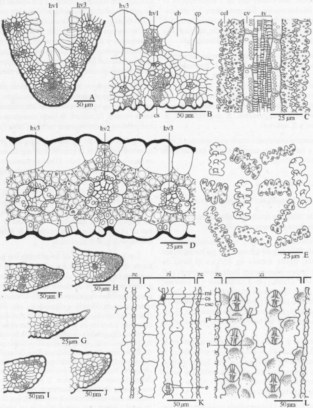
Fig. 2. Dibujos de transcortes y epidermis foliar con MO. A, detalle de la zona de la quilla o vena media en Schizachyrium bimucronatum (Peichoto 12); B, detalle de la porción media de la hemilamina en S. tenerum (Peichoto & Schinini 9), C, D y E, S. scabriflorum (Vanni et al. 4603) C, vista paradermal de un haz vascular con las células clorénquimáticas adyacentes, D, detalle de la disposición de las células del clorénquima en relación a los haces vasculares, en transcorte; E, células del clorénquima aisladas en corte longitudinal y en esquema tridimensional; F, G, H, I y J, detalle de los márgenes foliares en transcorte: F, S. bimucronatum (Peichoto 12); G, S. lactiflorum (Arbo et al. 8829); H, S. microstachyum ssp. microstachyum (Peichoto 11); I, S. sanguineum (Peichoto & Schinini 7); J, S. tenerum (Peichoto & Schinini 9). K y L, vista superficial de la epidermis de S. brevifolium (Sulekic 816), K, epidermis adaxial; L, epidermis abaxial. Abreviaturas: hv1: haz vascular de primer orden, hv2: haz vascular de segundo orden, hv3: haz vascular de tercer orden, cb: célula buliforme, cp: célula parenquimática, p: papilas, cs: célula silícica, tv: tejido vascular, cv: célula de la vaina vascular, ccl: célula del clorénquima, zc: zona costal, zi: zona intercostal, mi: micropelo, es: estoma, csc: cuerpo silíceo costal, pi: papila interestomática.
