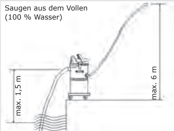
Schlürfbetrieb (Wasser-Luft-Gemisch)
