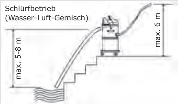
Förderweite
